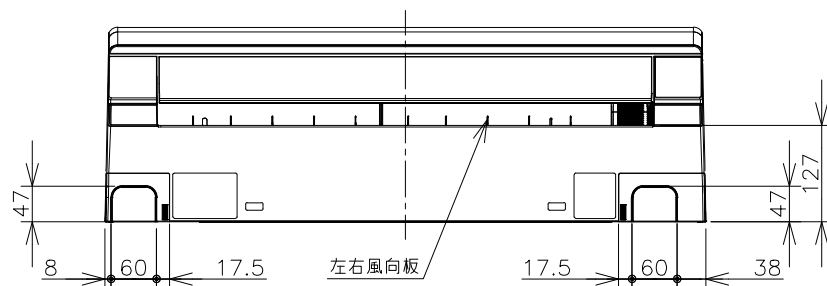
背面図
