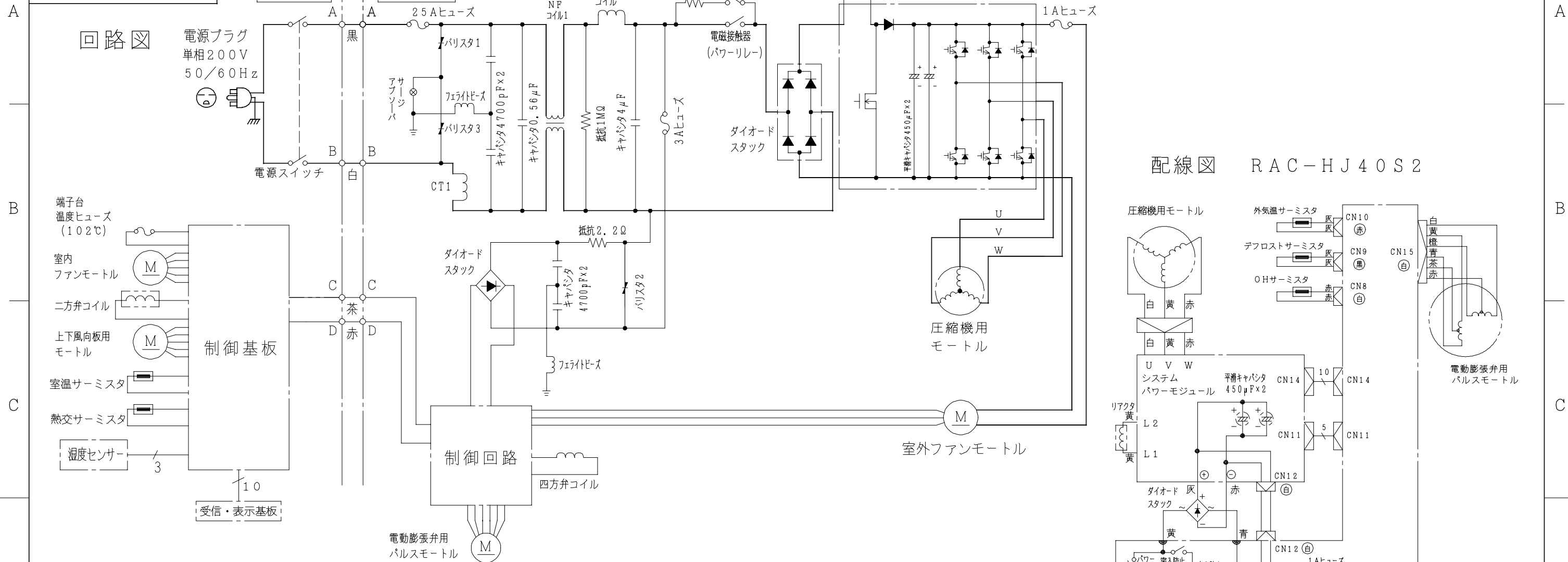
配線図
