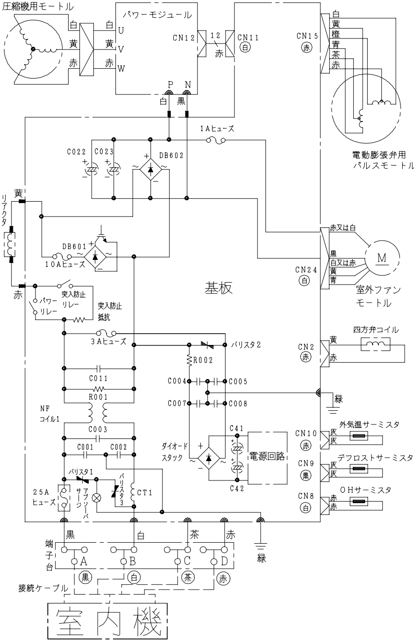
配線図 RAC-G50V2
