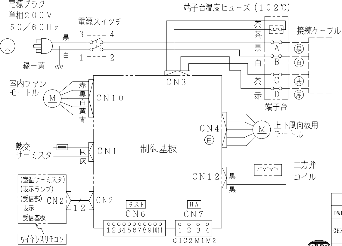
配線図 RAS-GZ50V2
