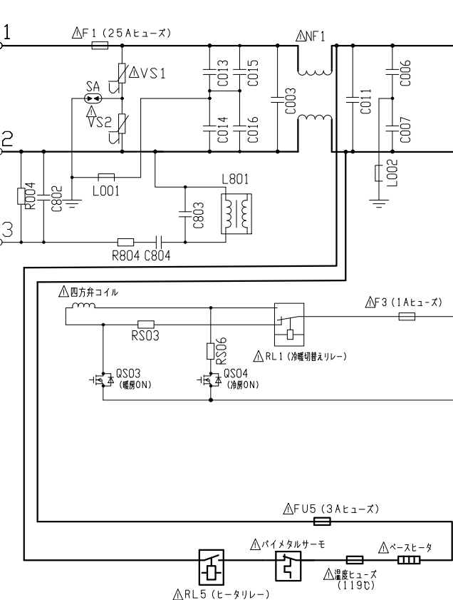
配線図 RAS-EK56L2
