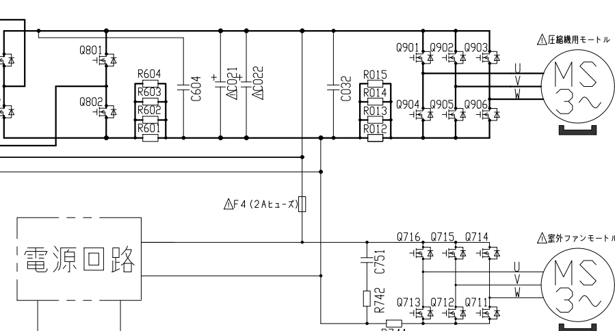
配線図 RAC-EK56L2
