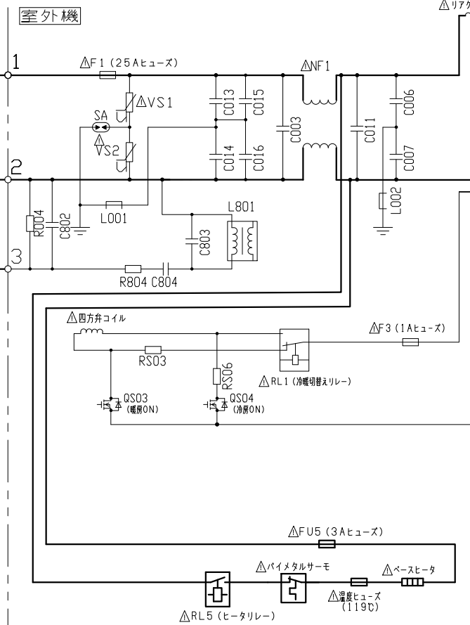
配線図 RAS-EK40L2
