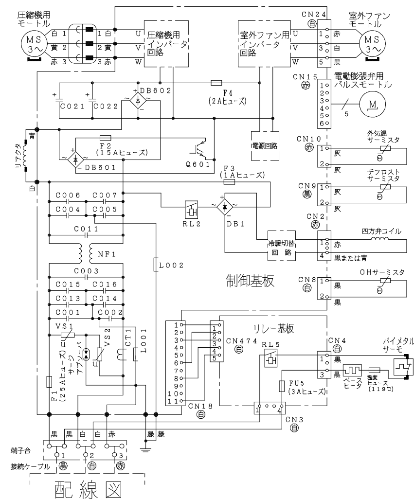
配線図 RAC-EK40J2
