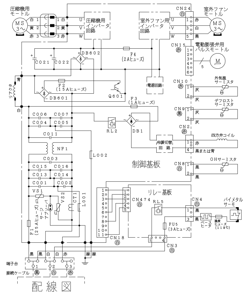
配線図 RAC-EK25H2
