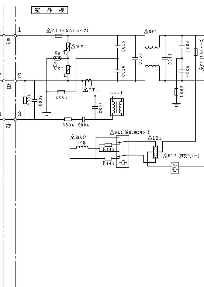
配線図 R A S - E B K 2 5 H
