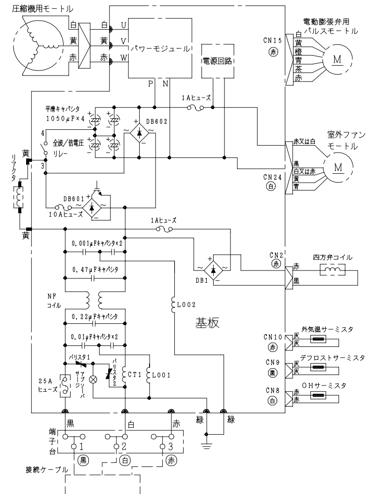
配線図 RAC-E28TE1
