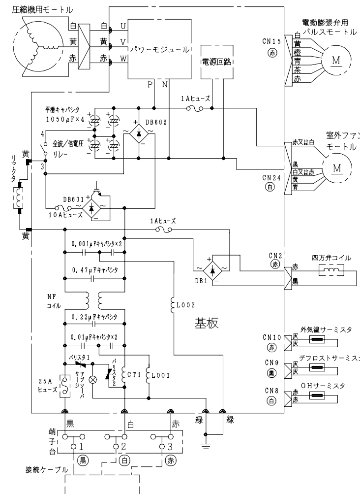
配線図 RAC-E25TE1
