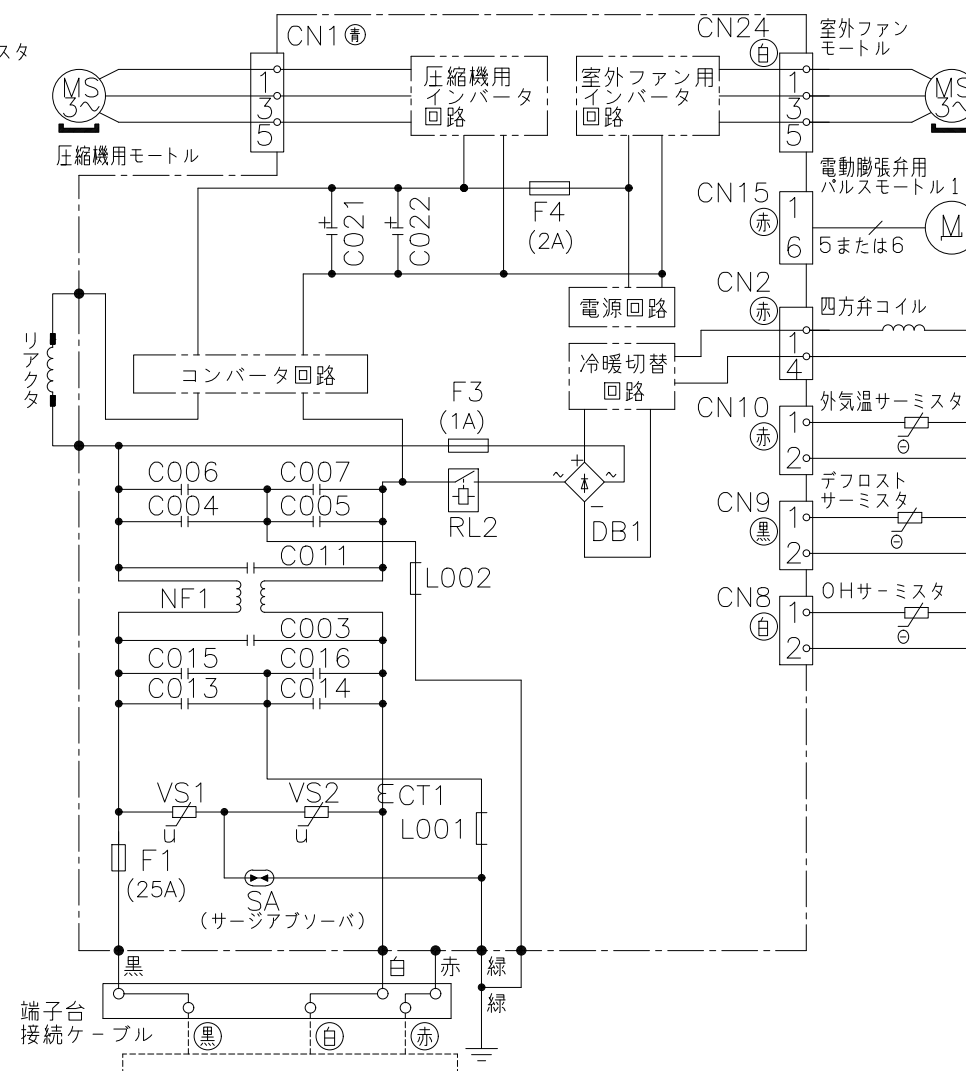
配線図 RAC-DT56K2
