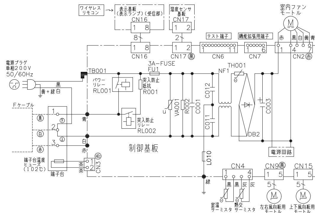
配線図 RAS-DT56K2
