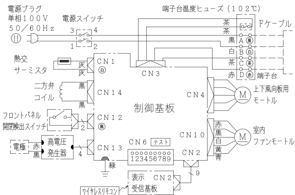
配線図 R A S - D 2 2 W E 4
