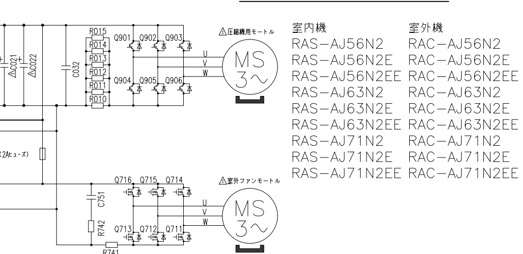
室外機配線図
