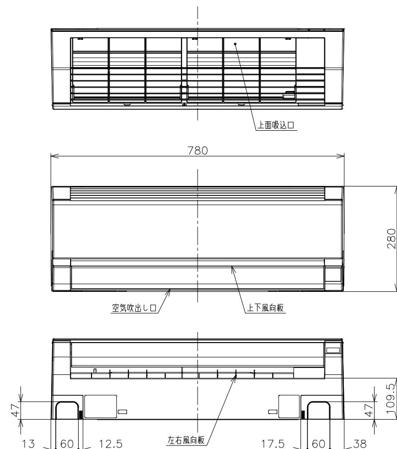
日立ルームエアコン 壁掛AJシリーズ室内ユニット寸法図
