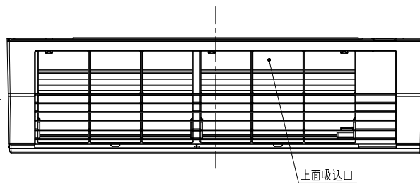
日立ルームエアコン 壁掛AJE, AJEEシリーズ室内ユニット寸法図
