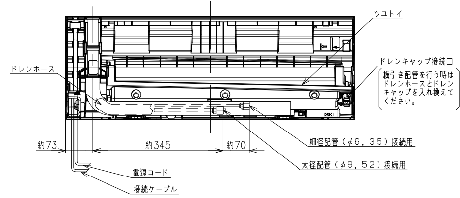
背面図
