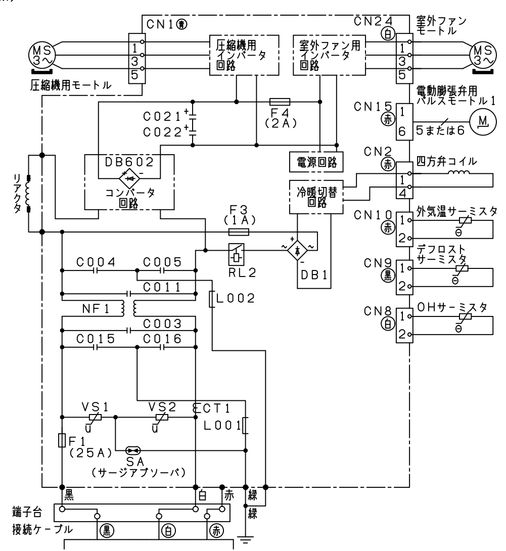
配線図 RAC-AJ40JE
