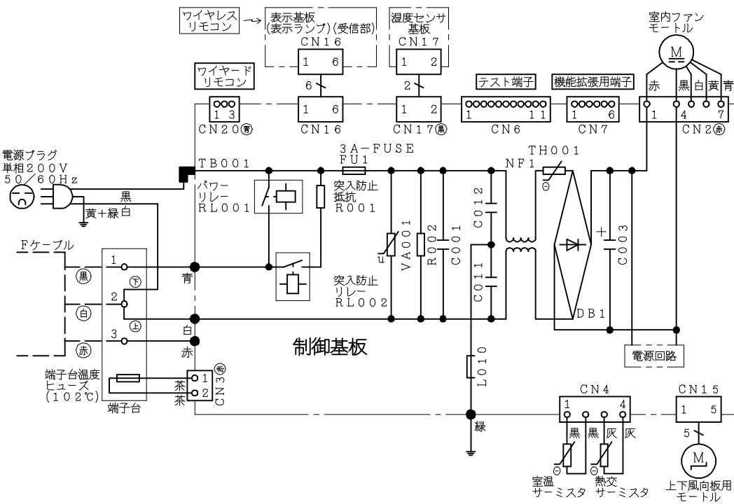
配線図 RAS-AJ40F2
