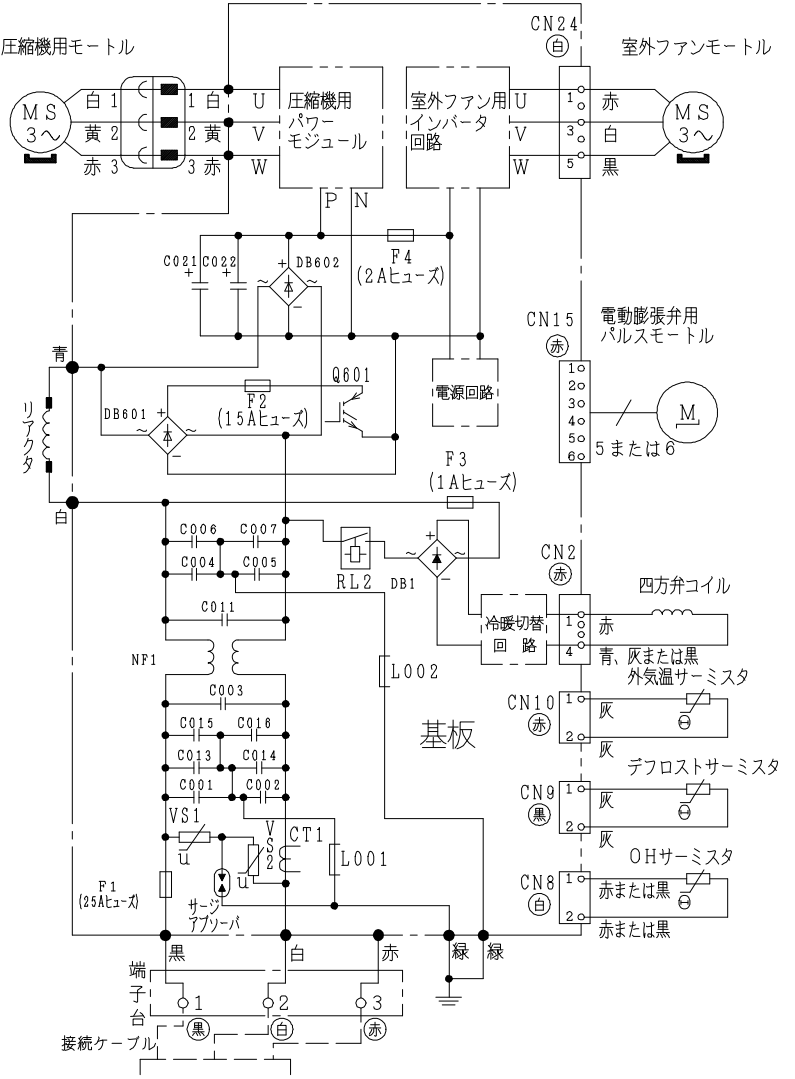
配線図 RAC-AJ40F2
