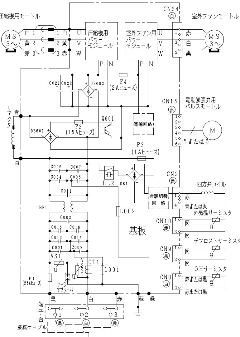
配線図 RAC-AJ40B2
