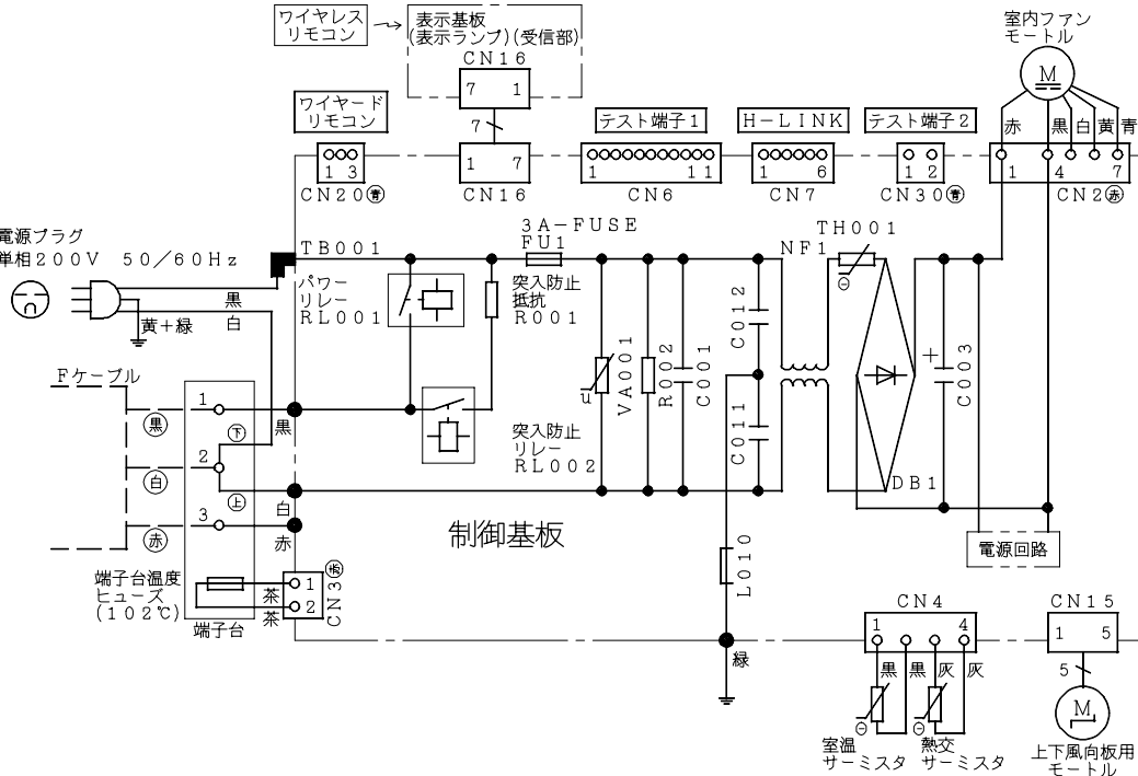
配線図 RAS-AJ40B2
