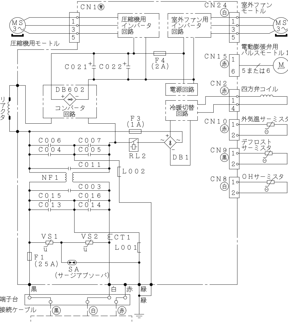
配線図 RAC-AJ36J2
