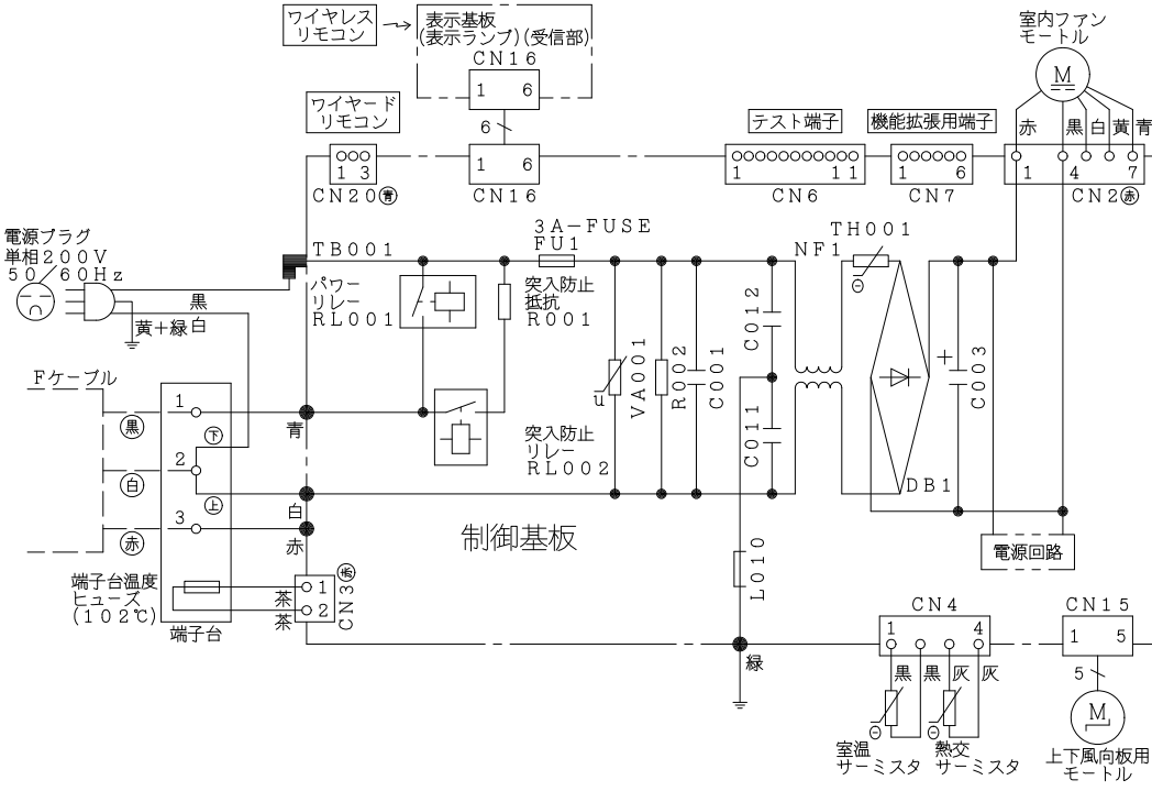
配線図 RAS-AJ36J2
