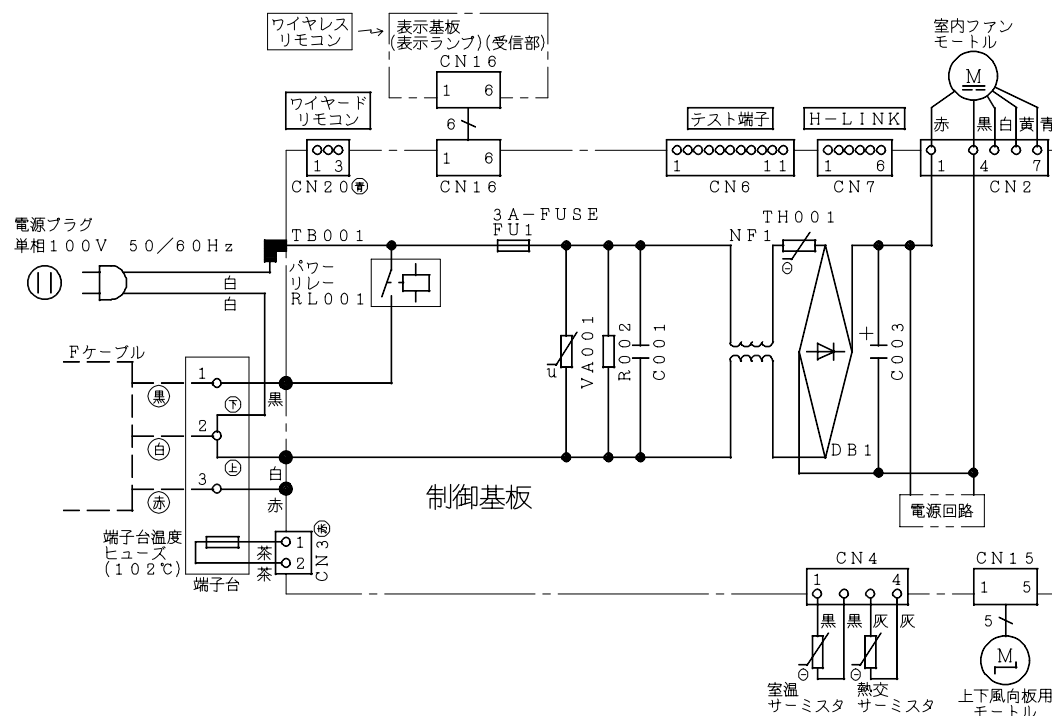
配線図 RAS-AJ36CE
