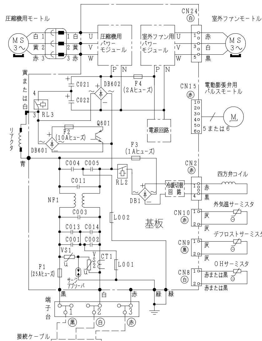
配線図 RAC-AJ36CE
