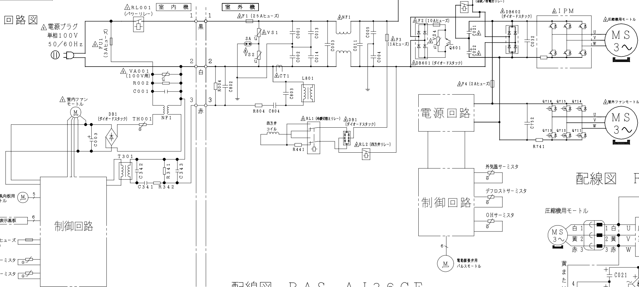
配線図 RAS-AJ36CE
