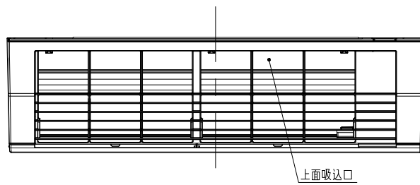
日立ルームエアコン 壁掛A Jシリーズ 室内ユニット寸法図
