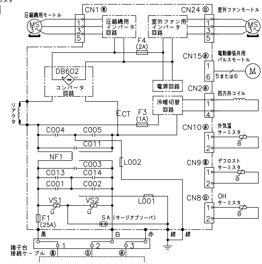
配線図 RAC-AJ25JE
