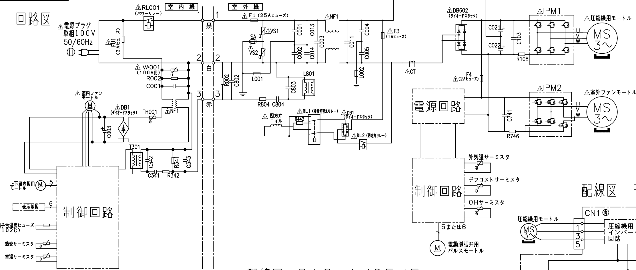
配線図 RAS-AJ25JE
