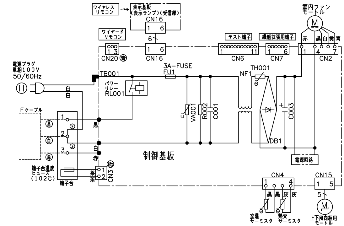
配線図 RAS-AJ25JE
