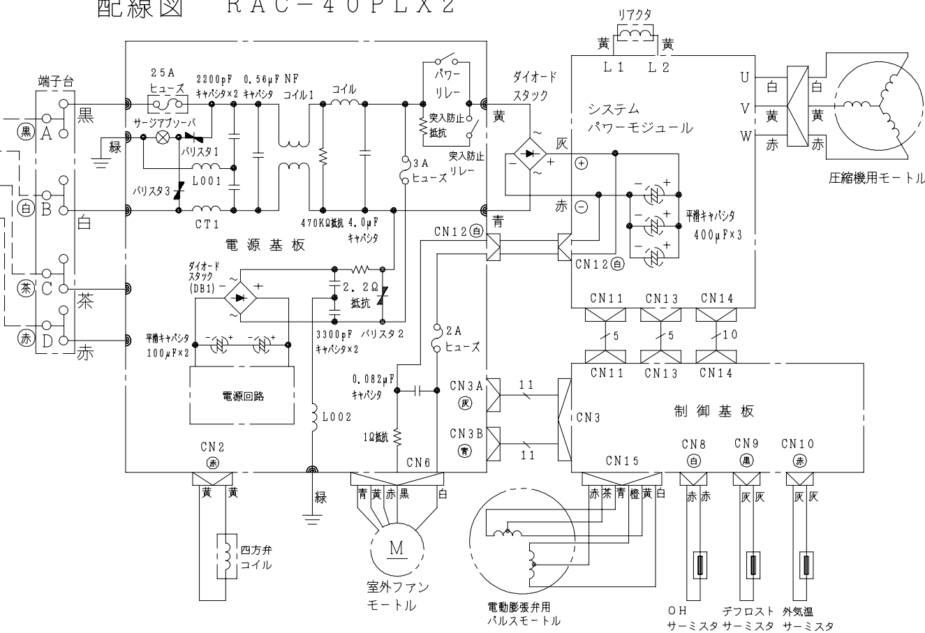
配線図 RAC-40PLX2
