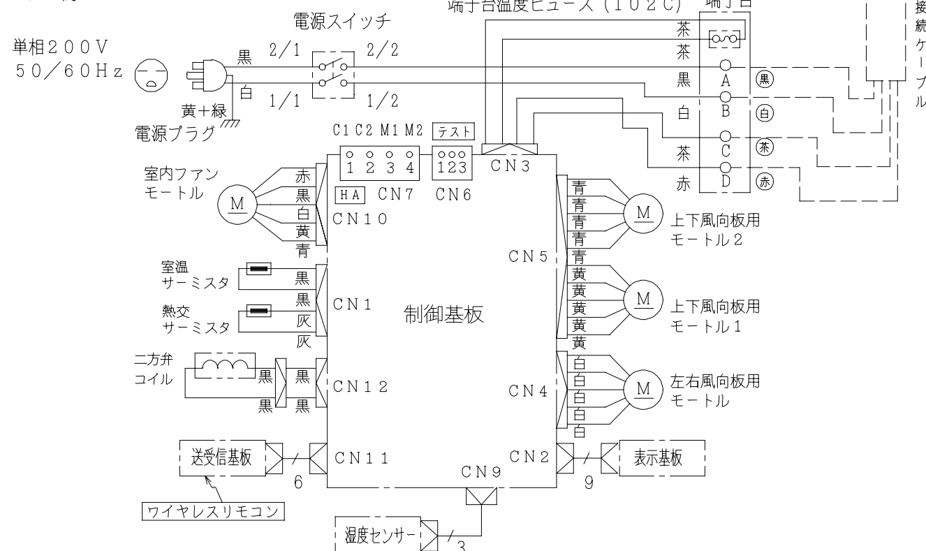
配線図 RAS-40PLX2
