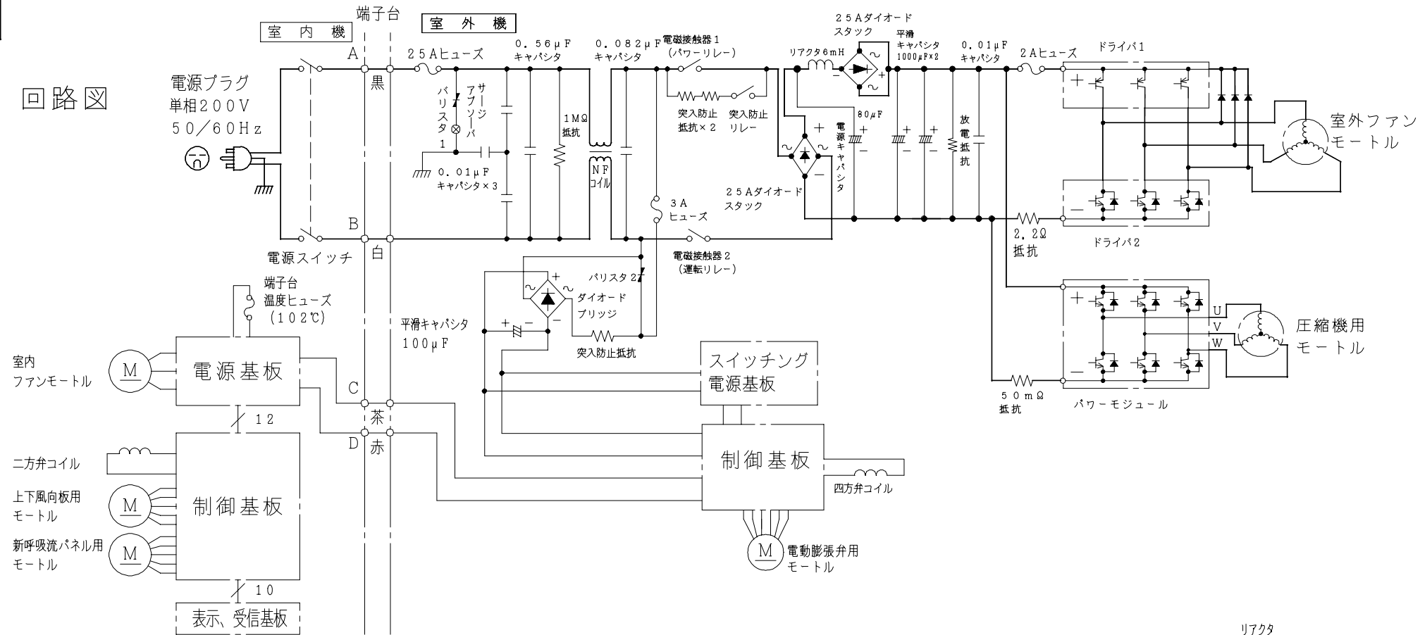
配線図 RAC-40HJX2
