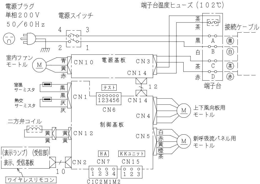
配線図 RAS-40HJX2
