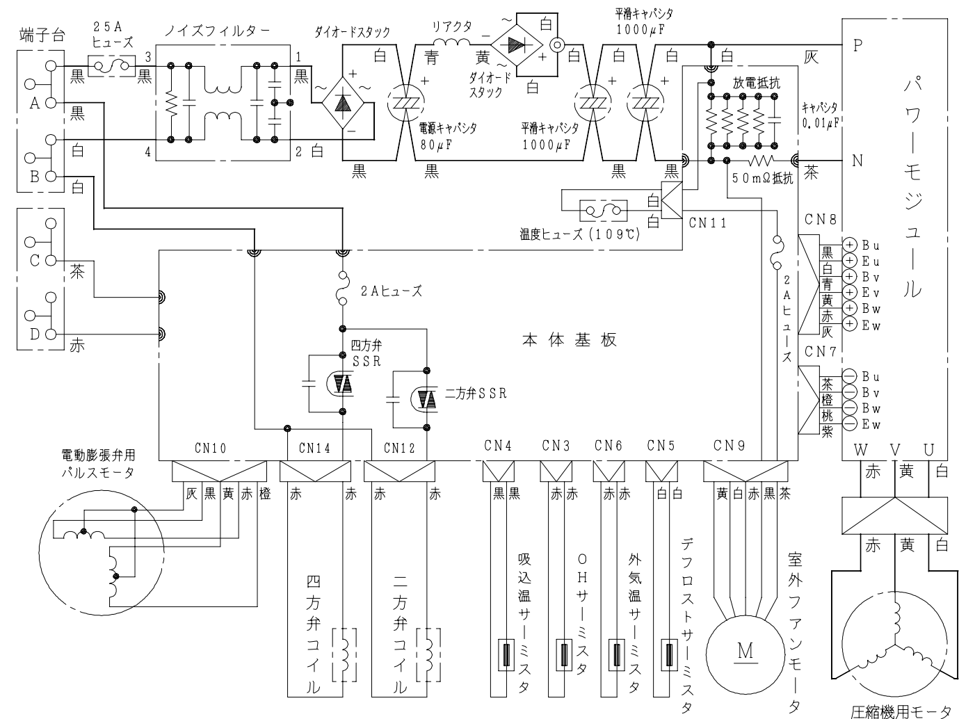
配線図 R A C - 4 0 F X 2 J K
