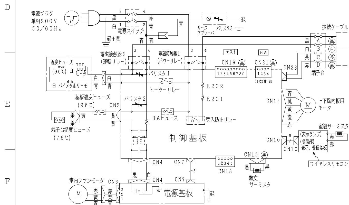
配線図 RAS-40FX2J
