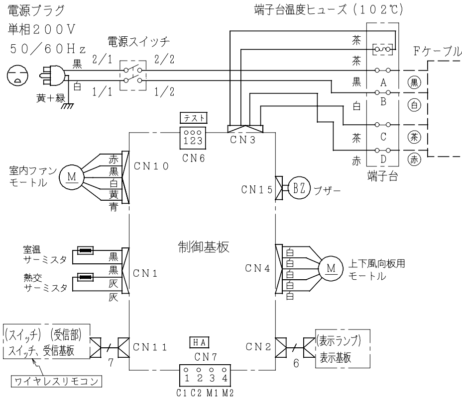
配線図 RAS-40FNX2
