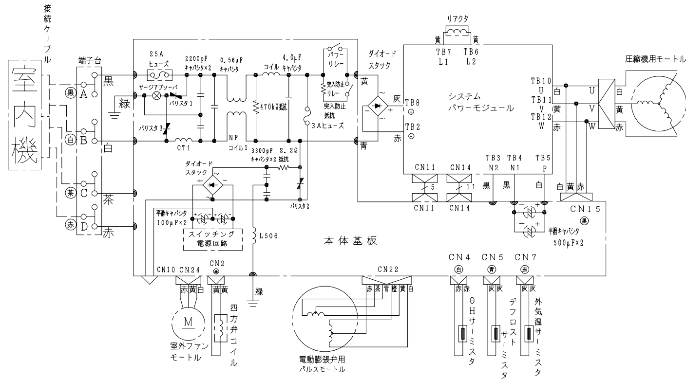
配線図 RAC-40FNX2
