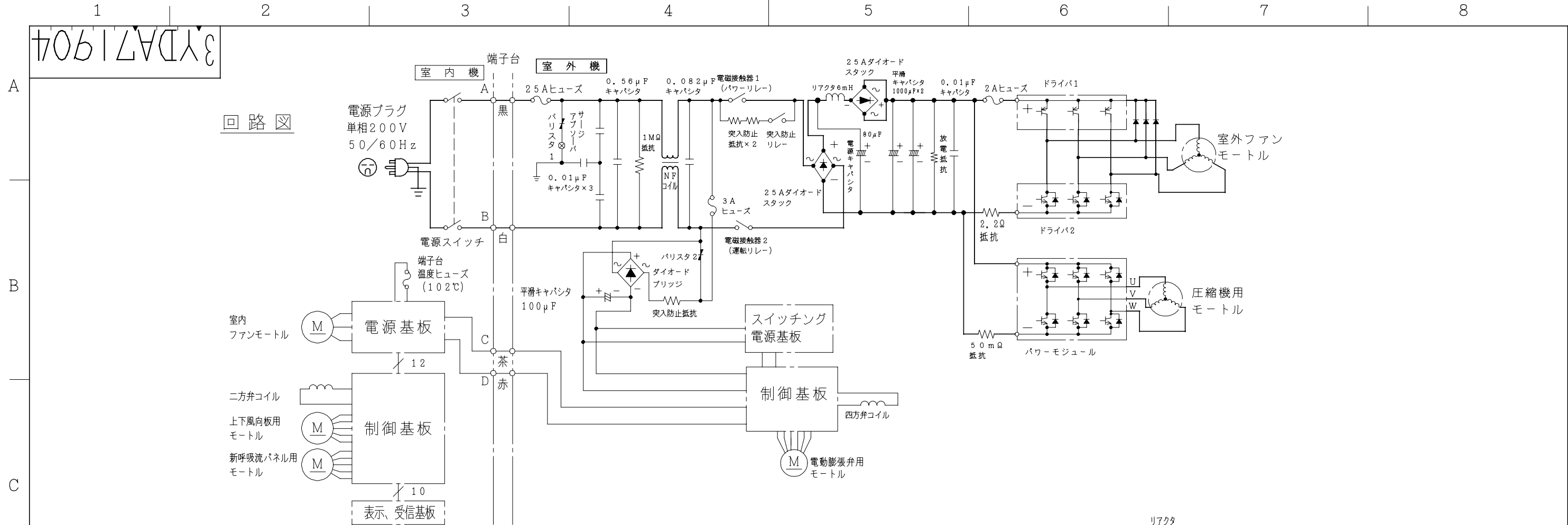
RAC-409GX2配線図
