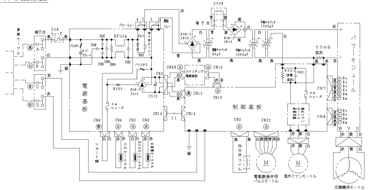
RAC-408GX2配線図
