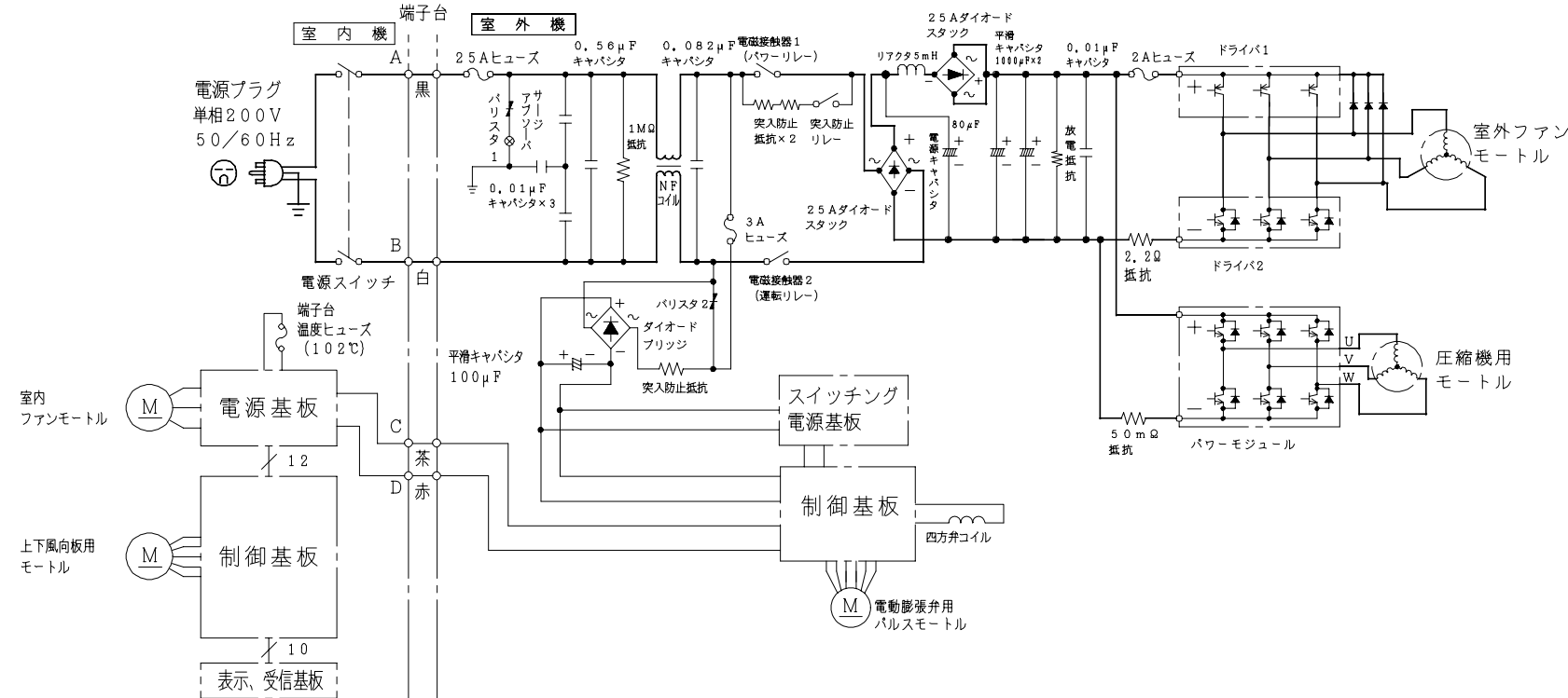
回路図
