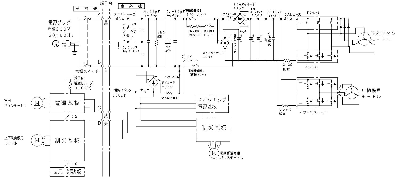
回路図
