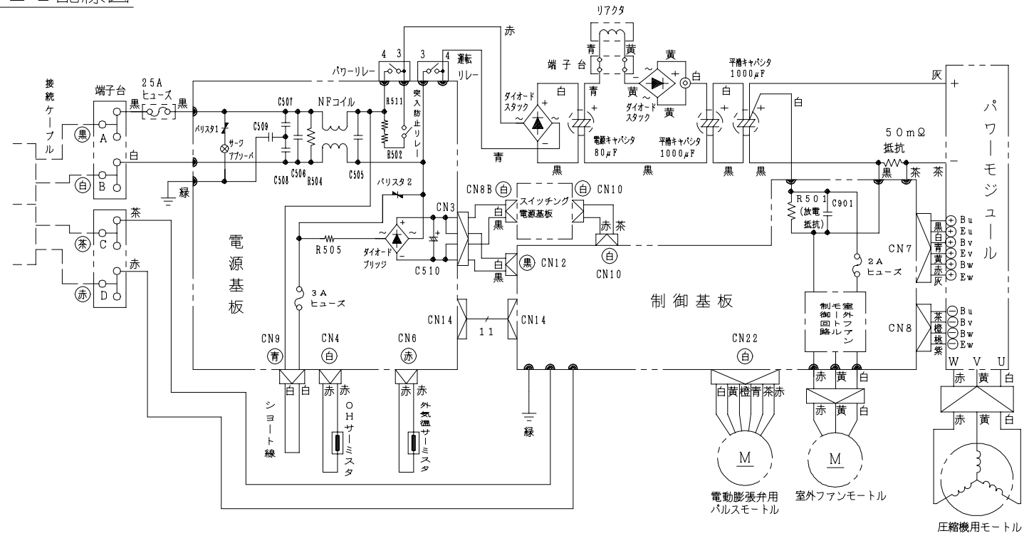
RAC-408GE2配線図
