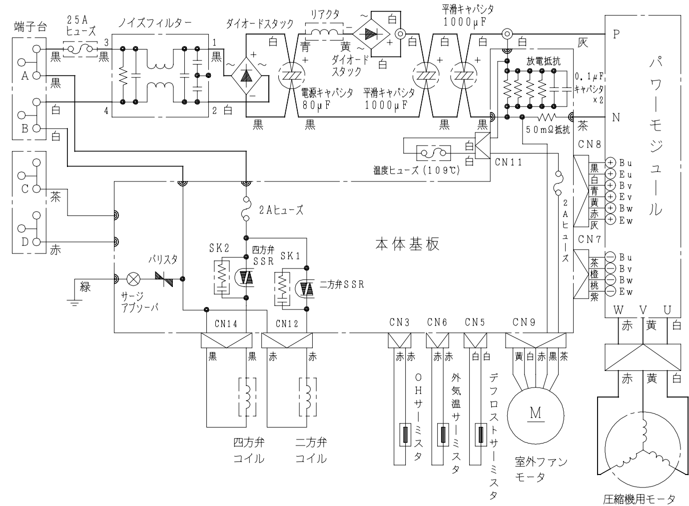
配線図 R A C - 3 2 9 D X 2
