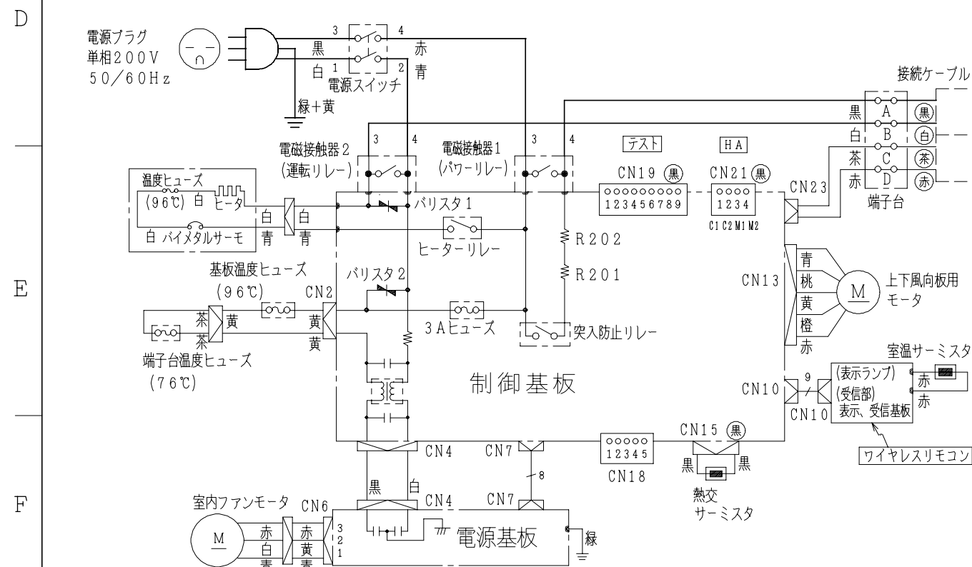
配線図 RAS-329DX2
