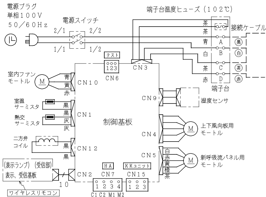
配線図 RAS-3210JX
