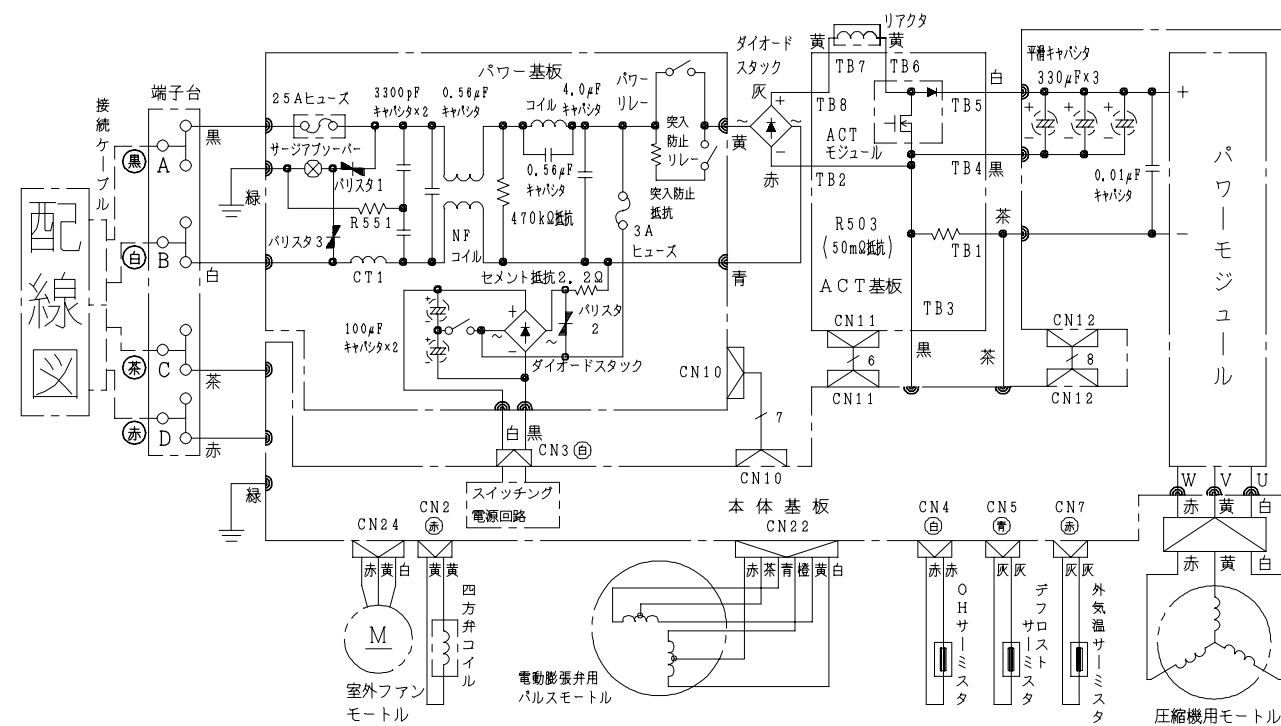
配線図 RAC-3210JX
