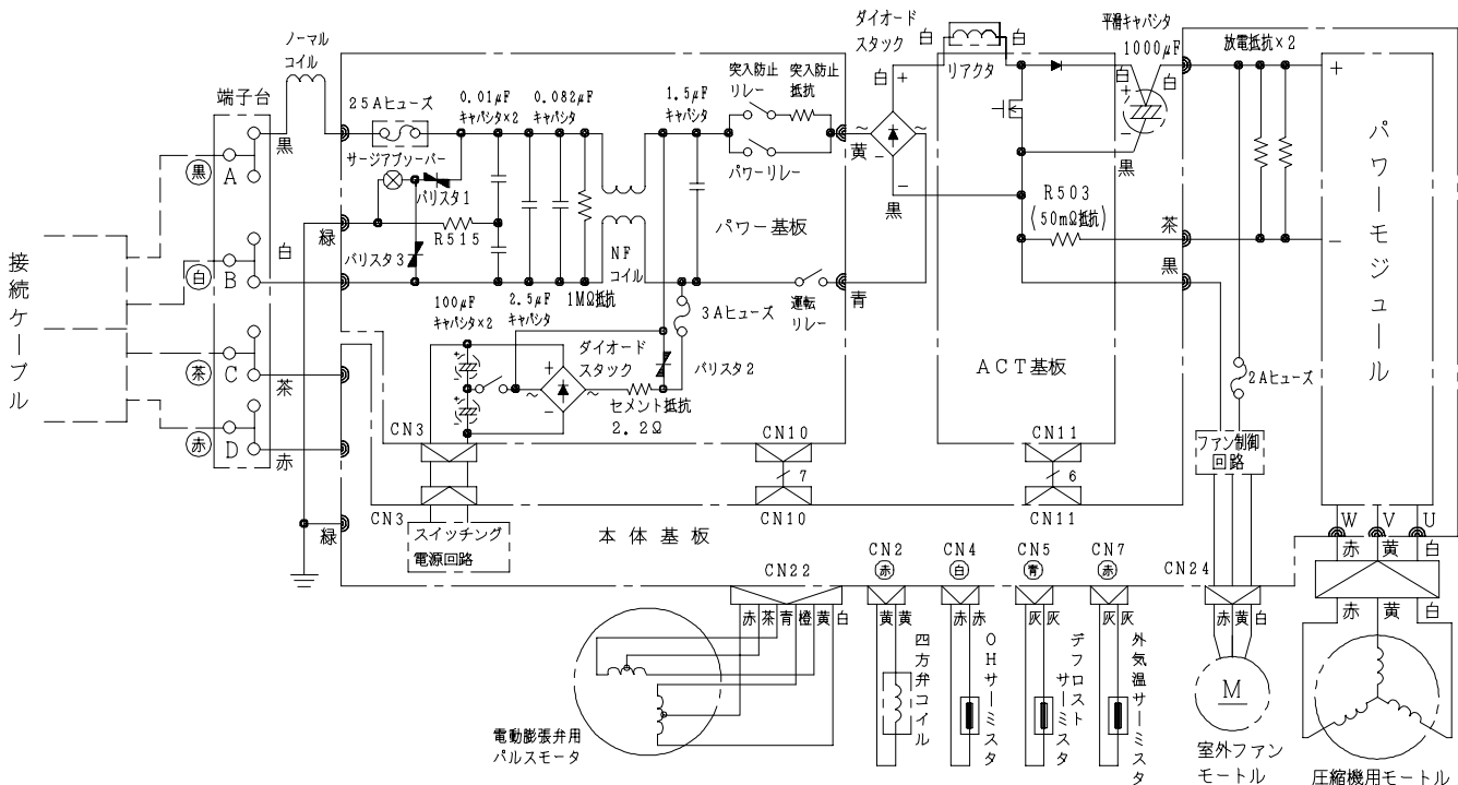
配線図 RAC-2810HX
