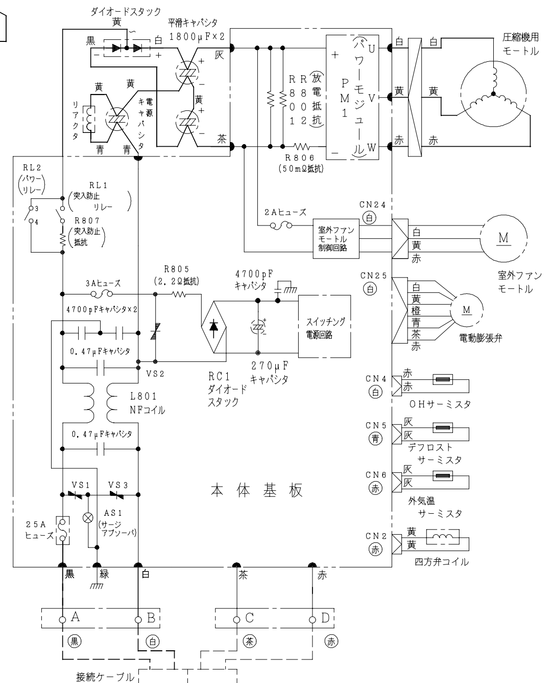
配線図 RAC-2809KX
