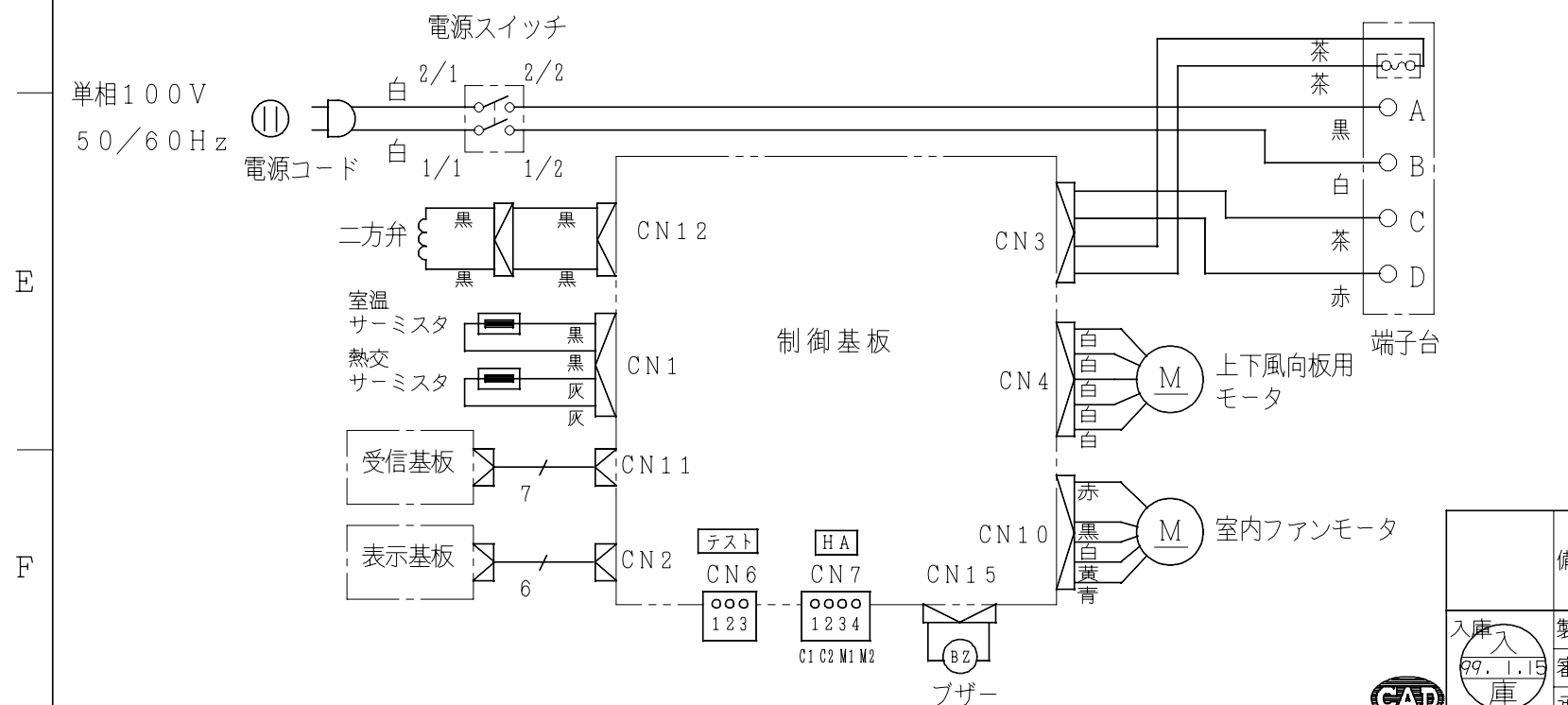
配線図 RAS-2809KX
