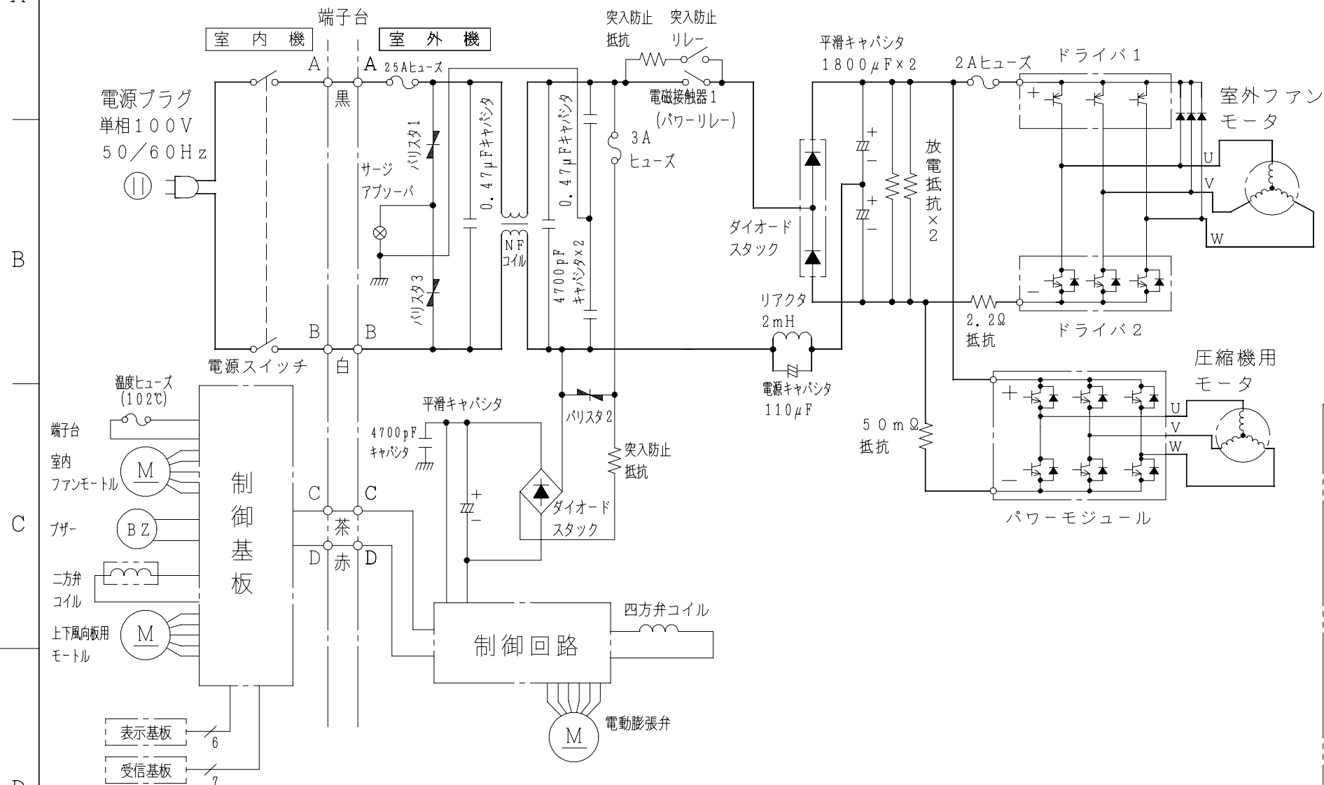
配線図 RAS-2809KX
