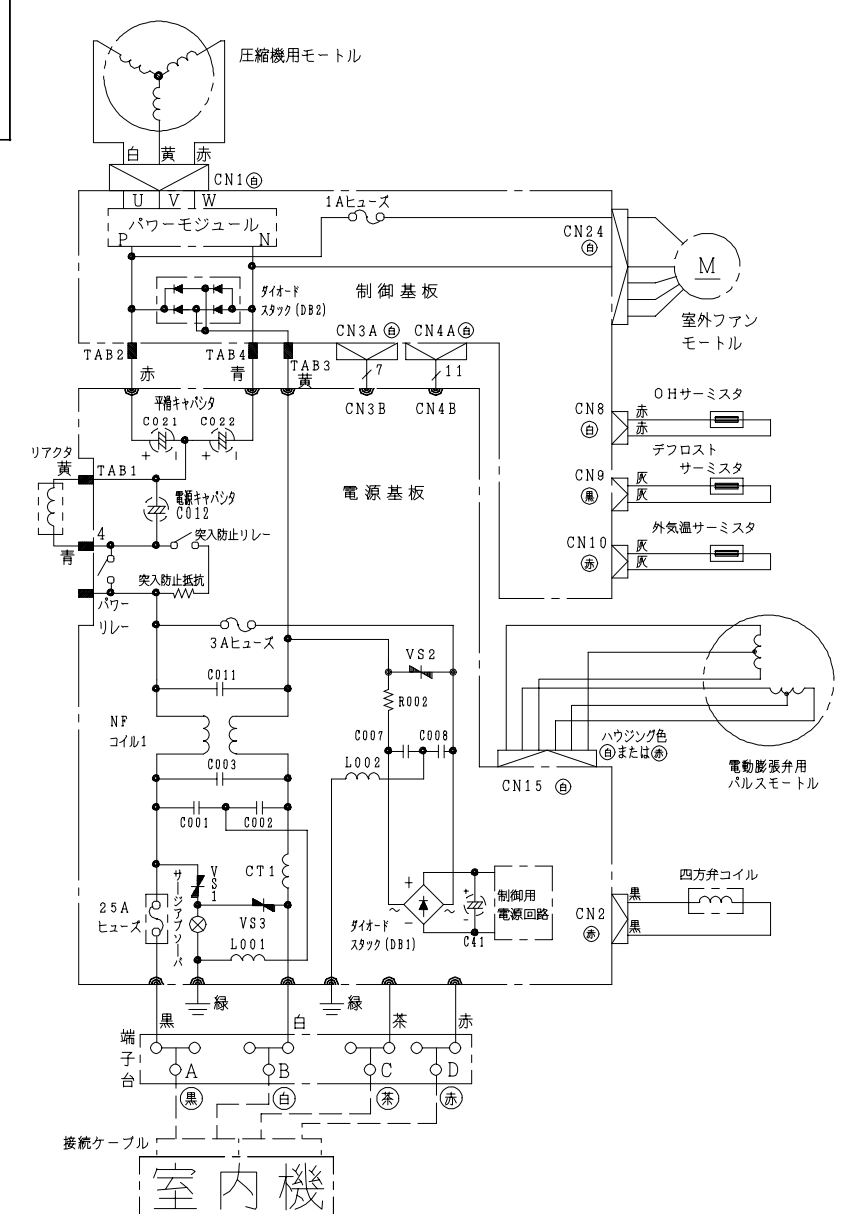
配線図 RAC-2800VJ
