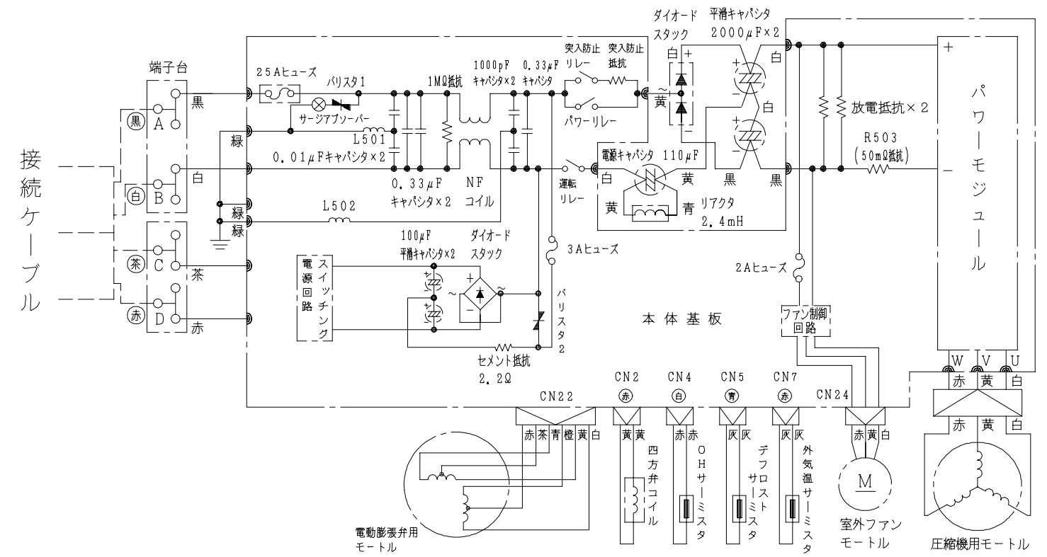
配線図 RAC-259HXD
