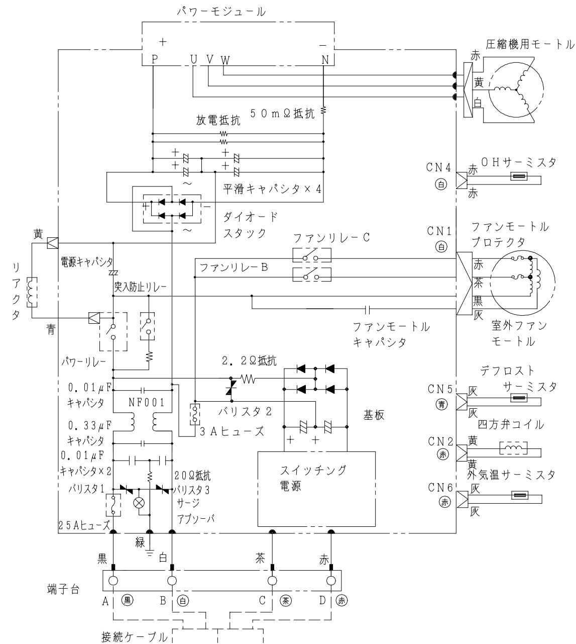
配線図 RAC-258JXD
