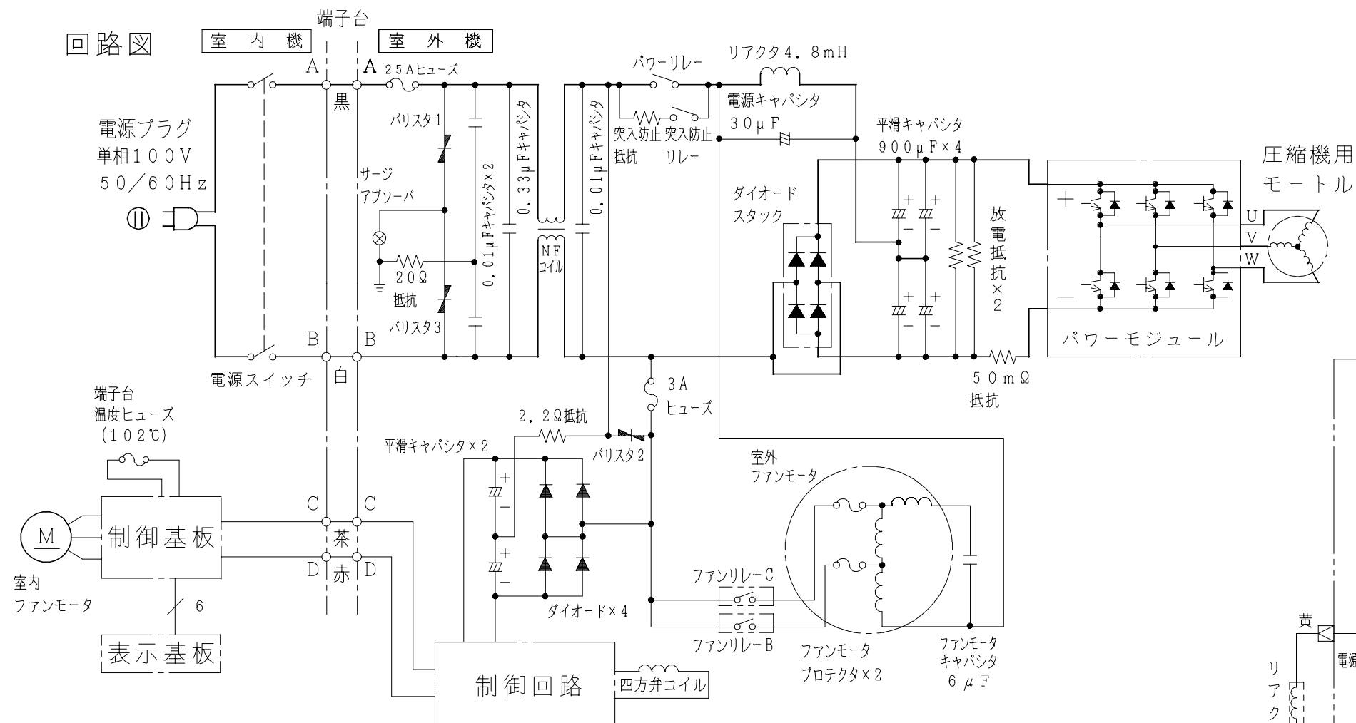
配線図 RAS-258JXD
