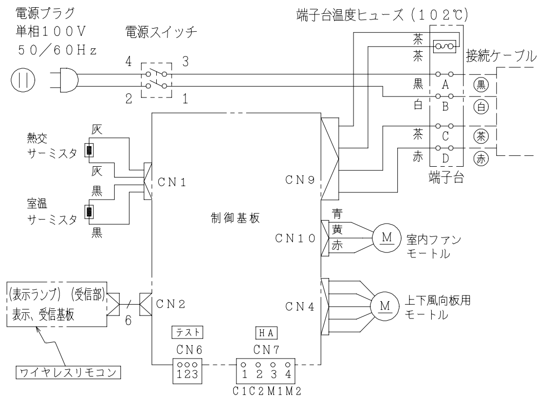
配線図 RAS-258JXD
