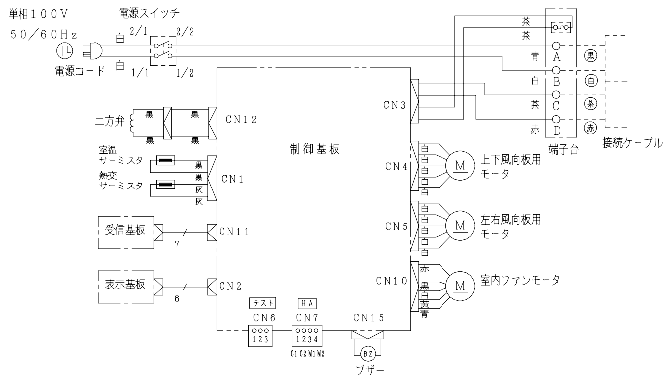
配線図 RAS-2511KX
