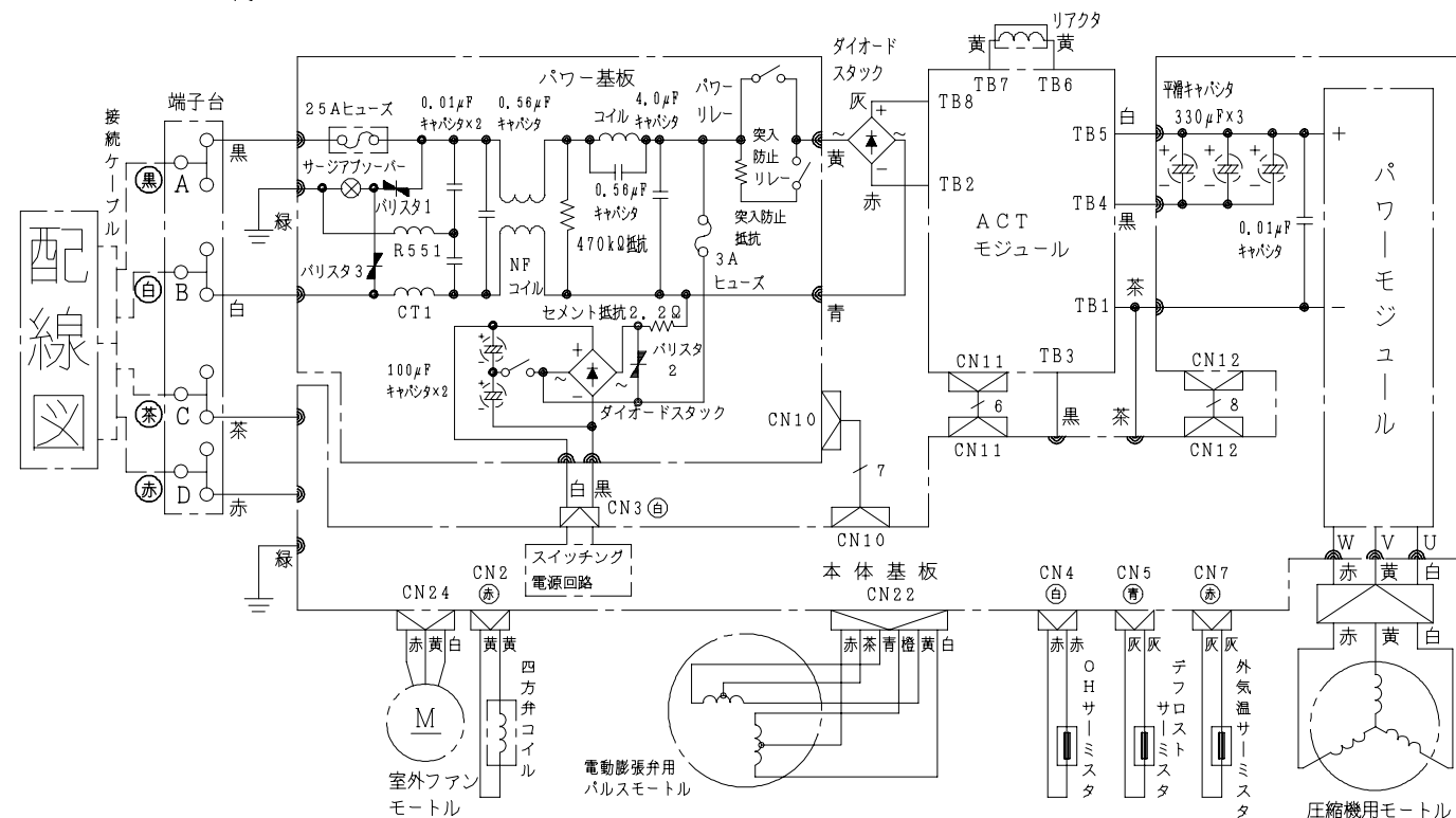
配線図 RAC-2510JX-1
