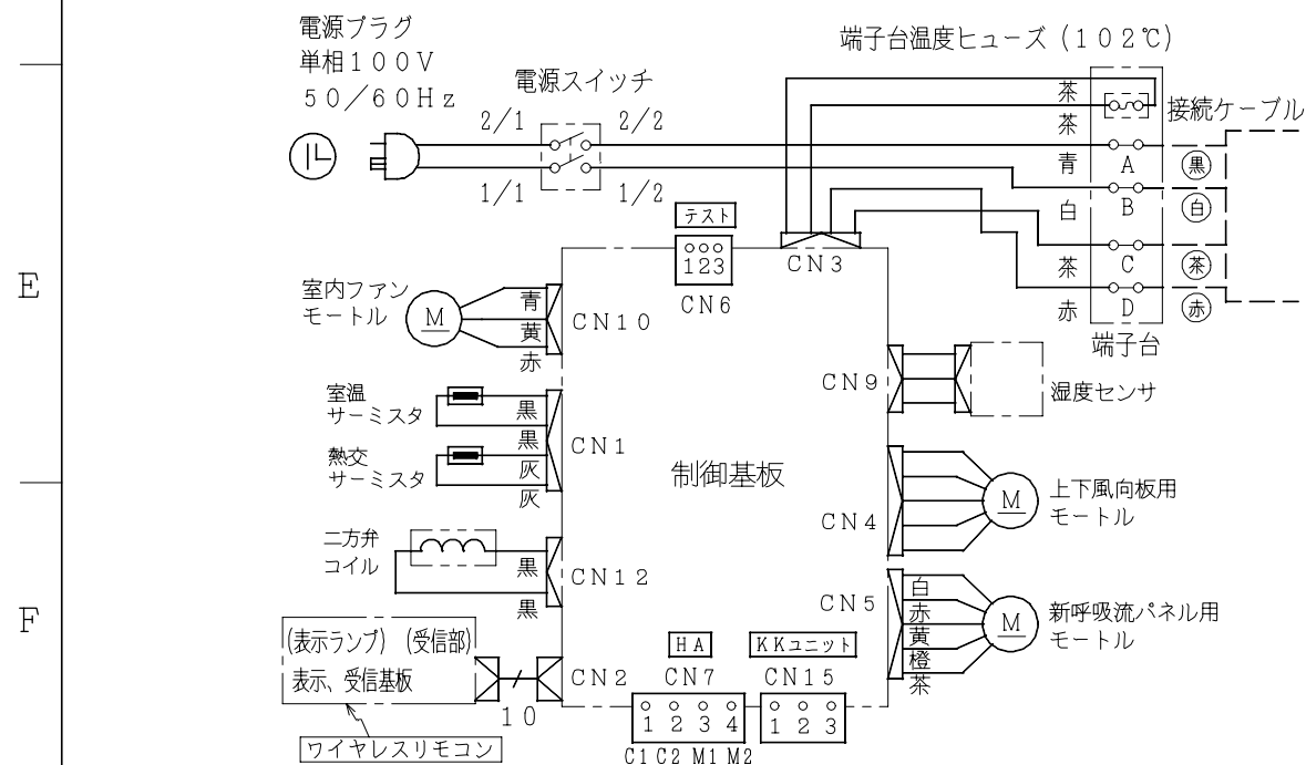
配線図 RAS-2510JX
