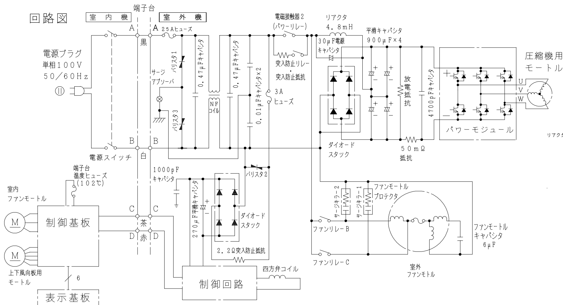
配線図 RAS-2508MX
