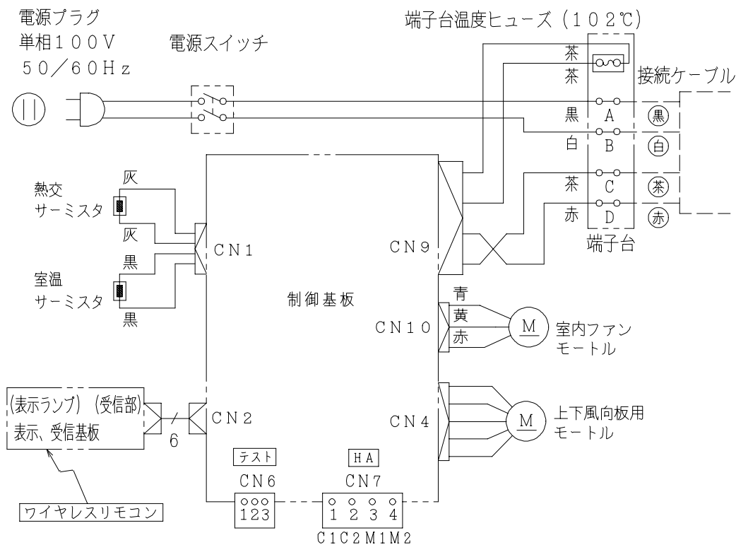
配線図 RAS-2508MX
