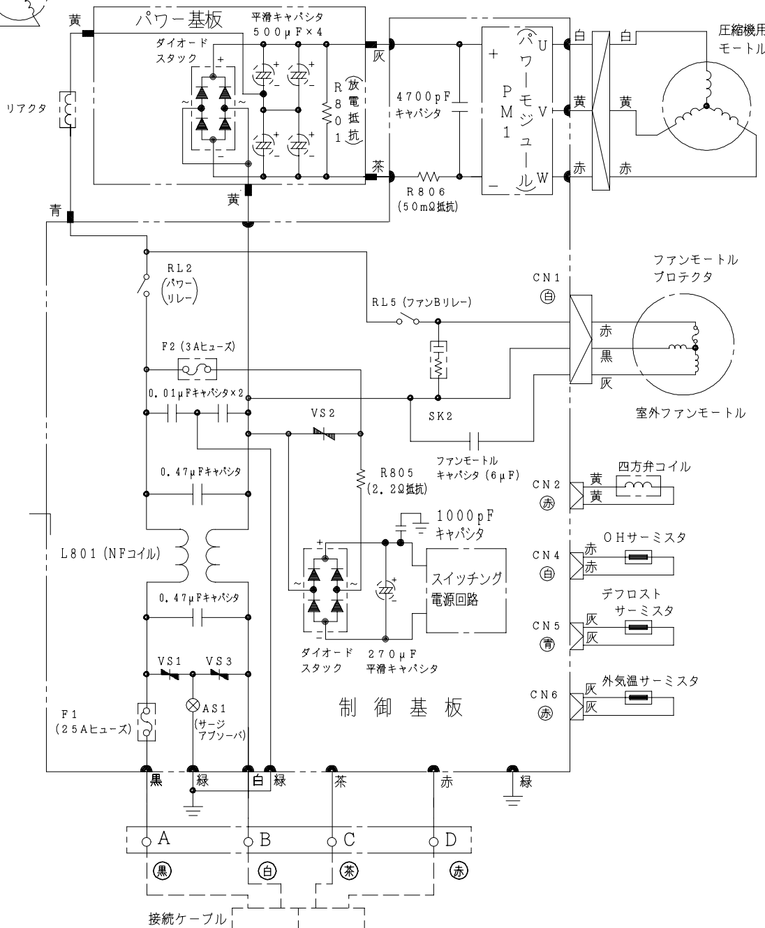
配線図 RAC-2208MX
