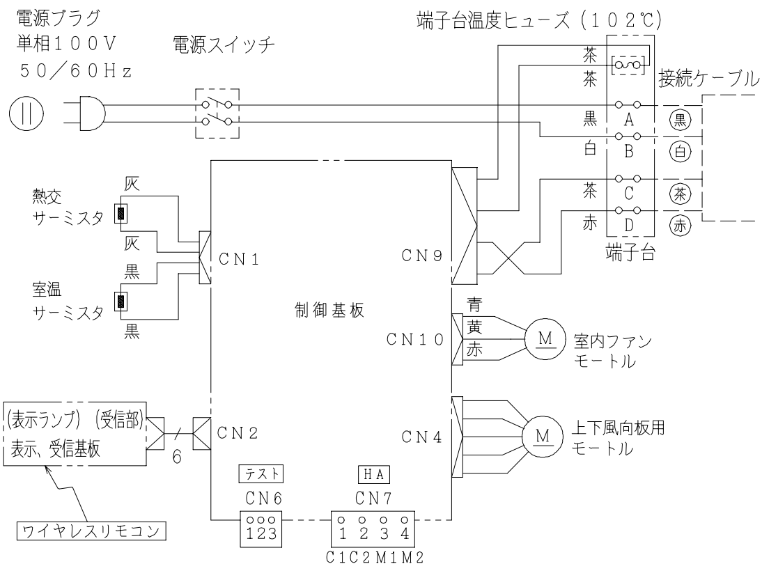
配線図 RAS-2208MX
