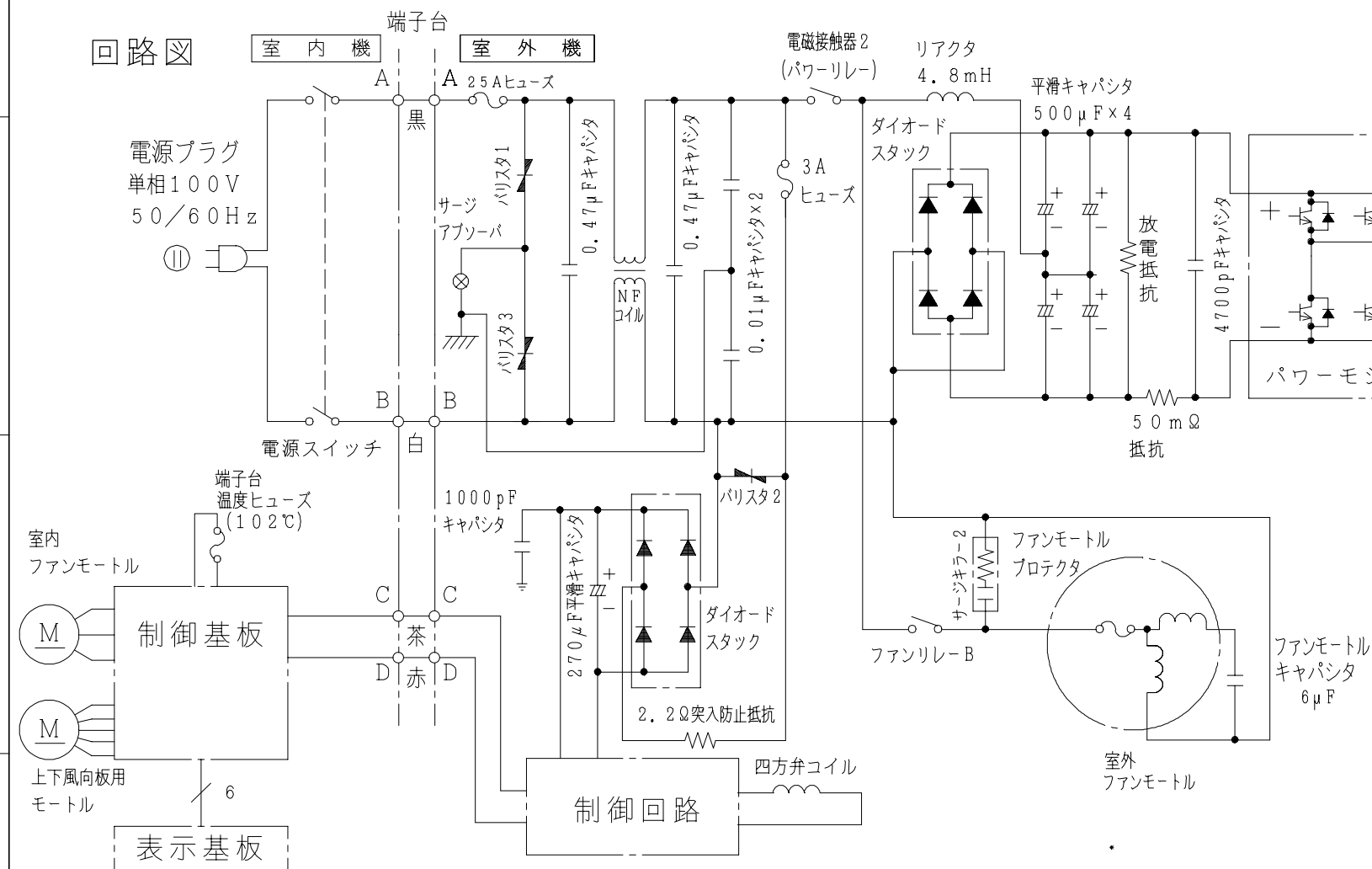
配線図 RAS-2208MX
