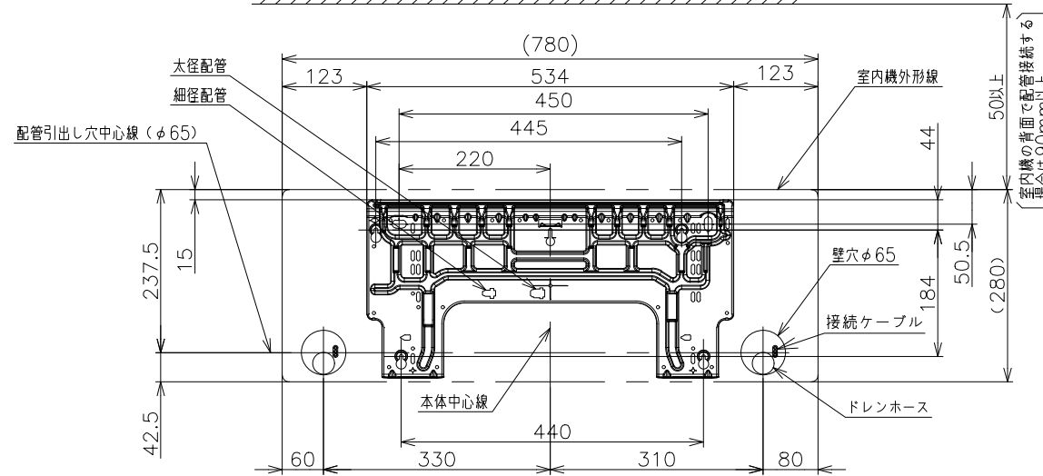
据付板
