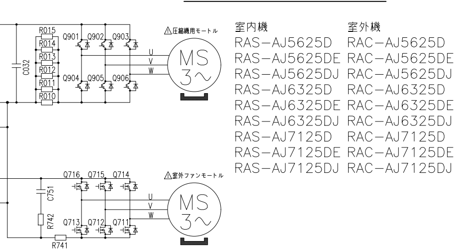
室外機配線図
