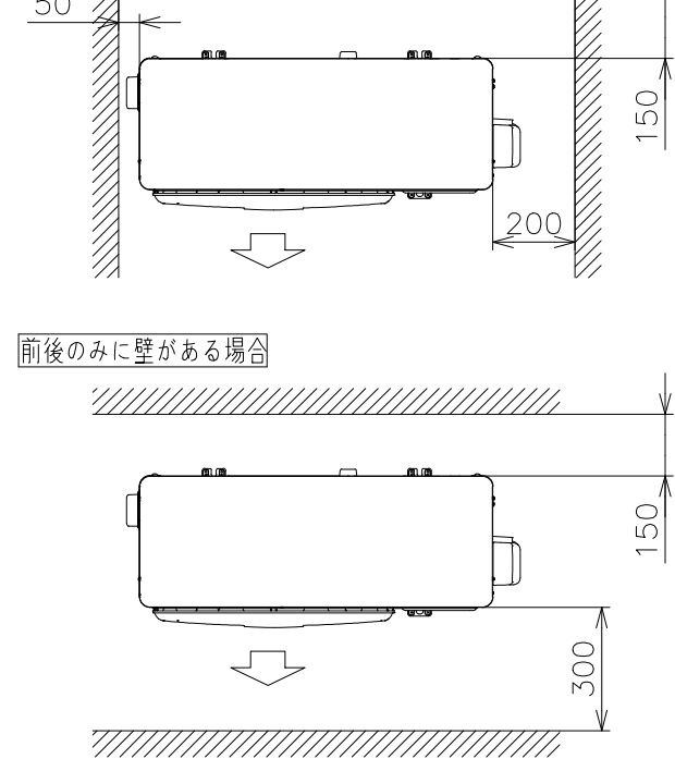
前後のみに壁がある場合
