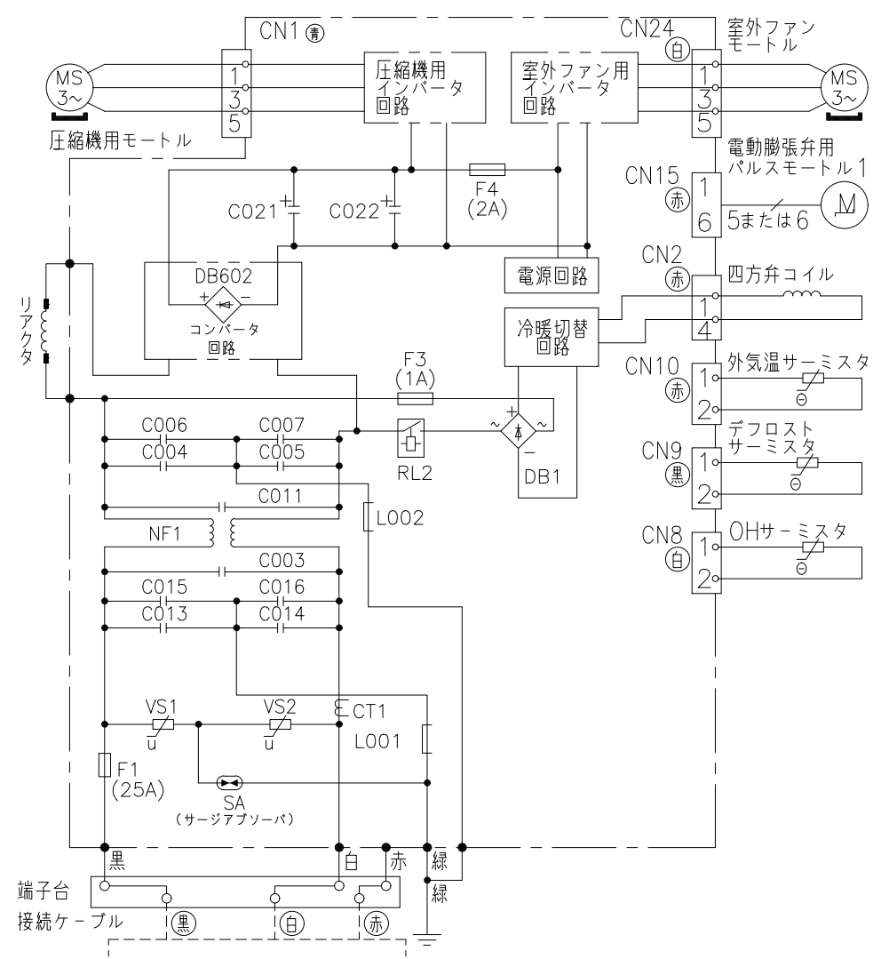
配線図 RAC-AJ36K2EE
