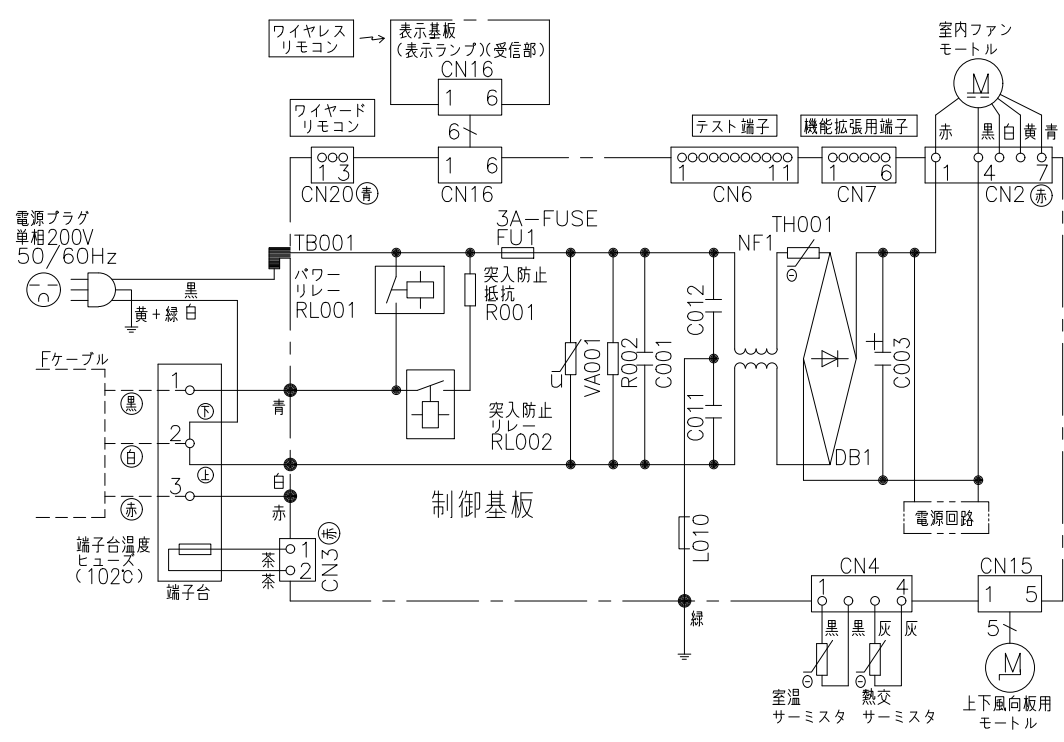
配線図 RAS-AJ36K2EE
