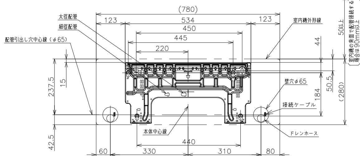
据付板
