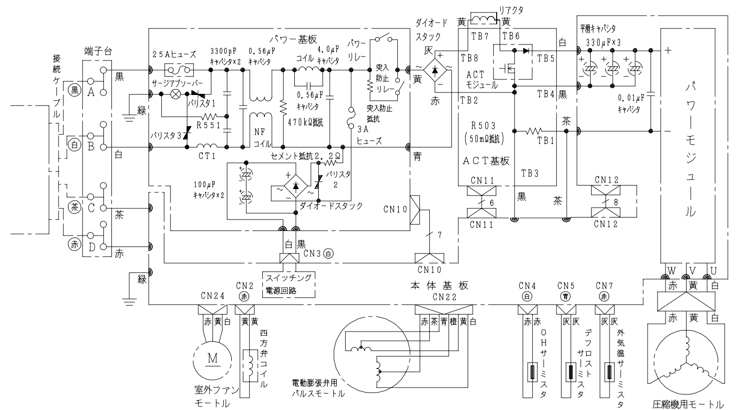
配線図 RAC-285JX2
