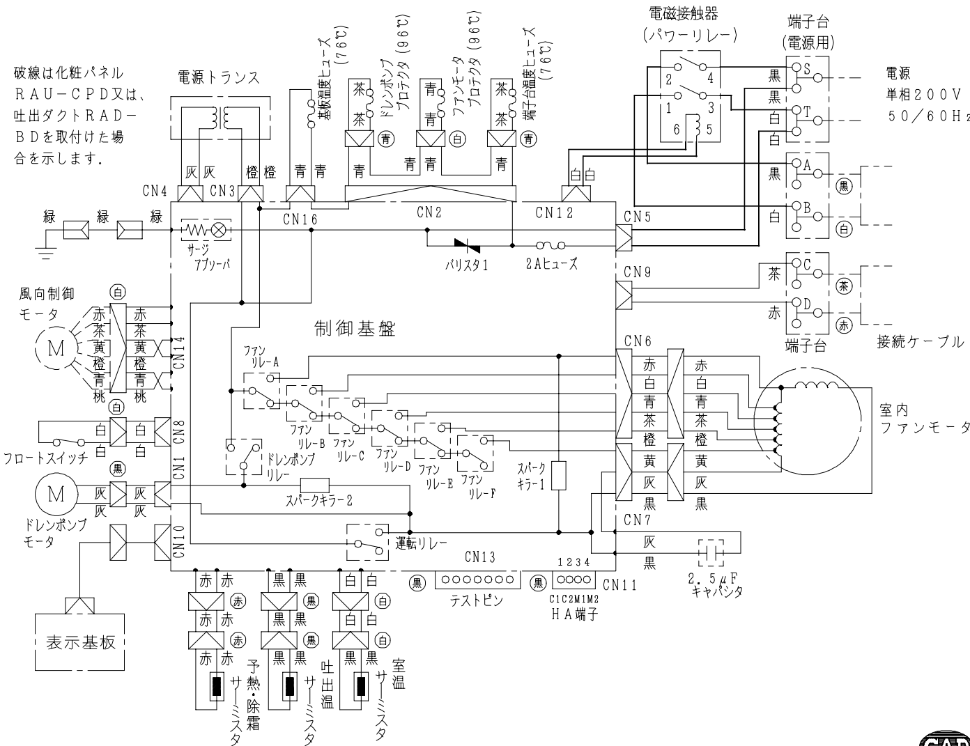
配線図 RAD-404DX2
