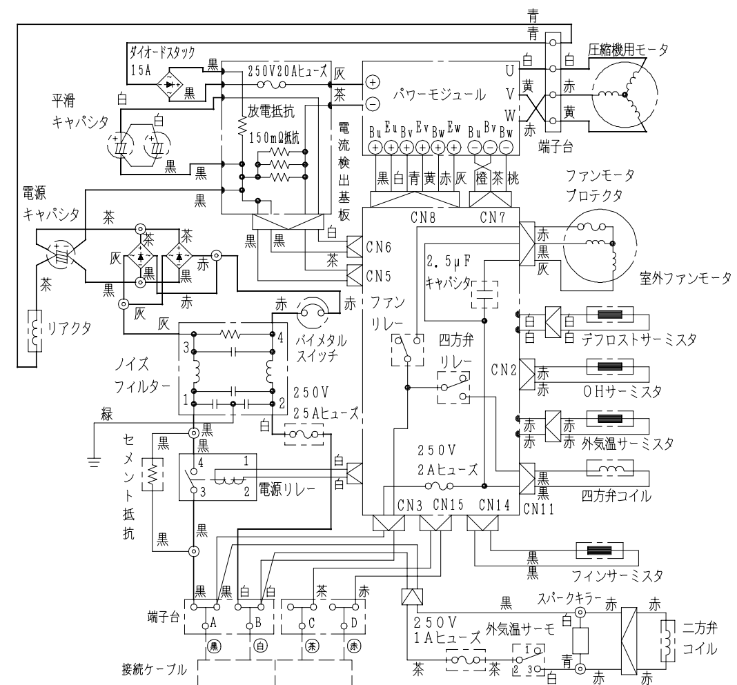
配線図 RAC-404DX2
