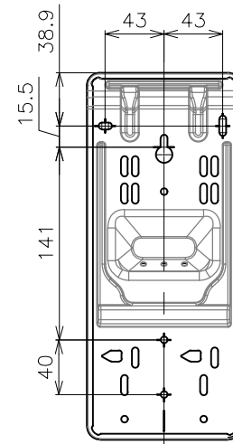
換気ユニット 据付穴位置
