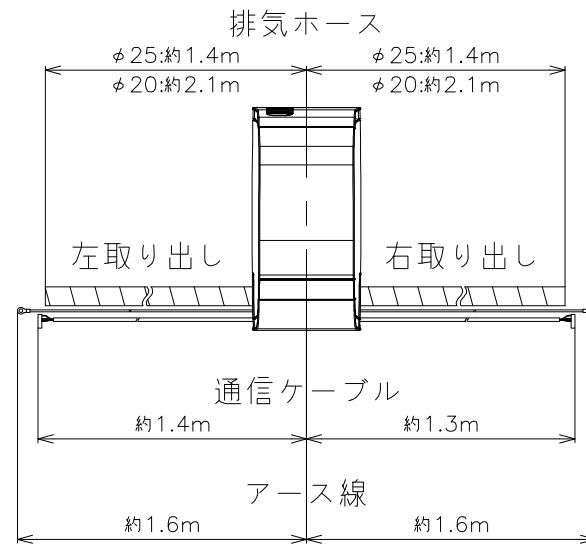
配線寸法
