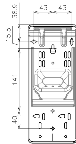
換気ユニット 据付穴位置
