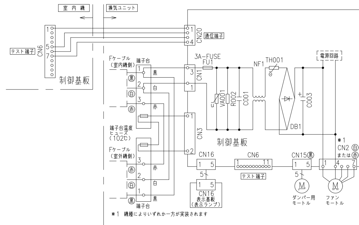
回路図
