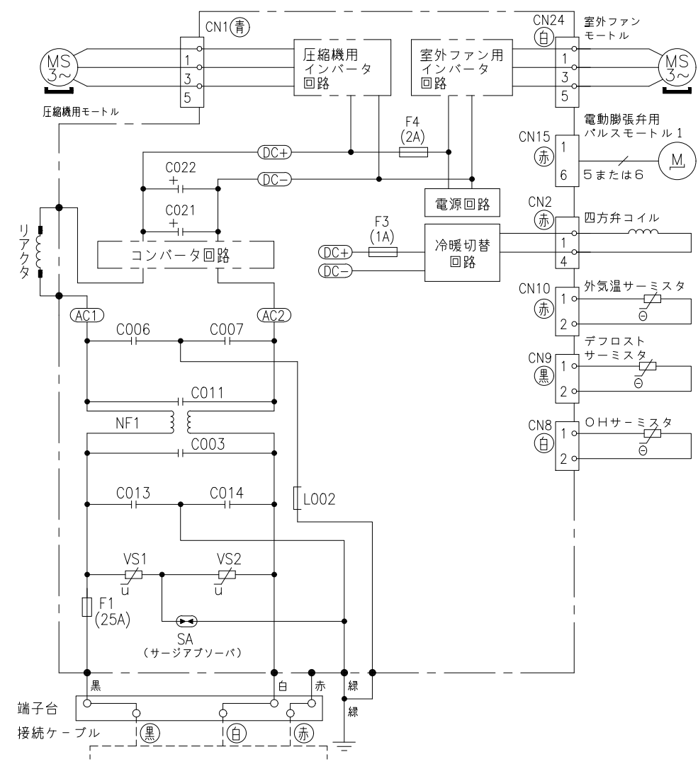
配線図 RAC-XJ56L2
