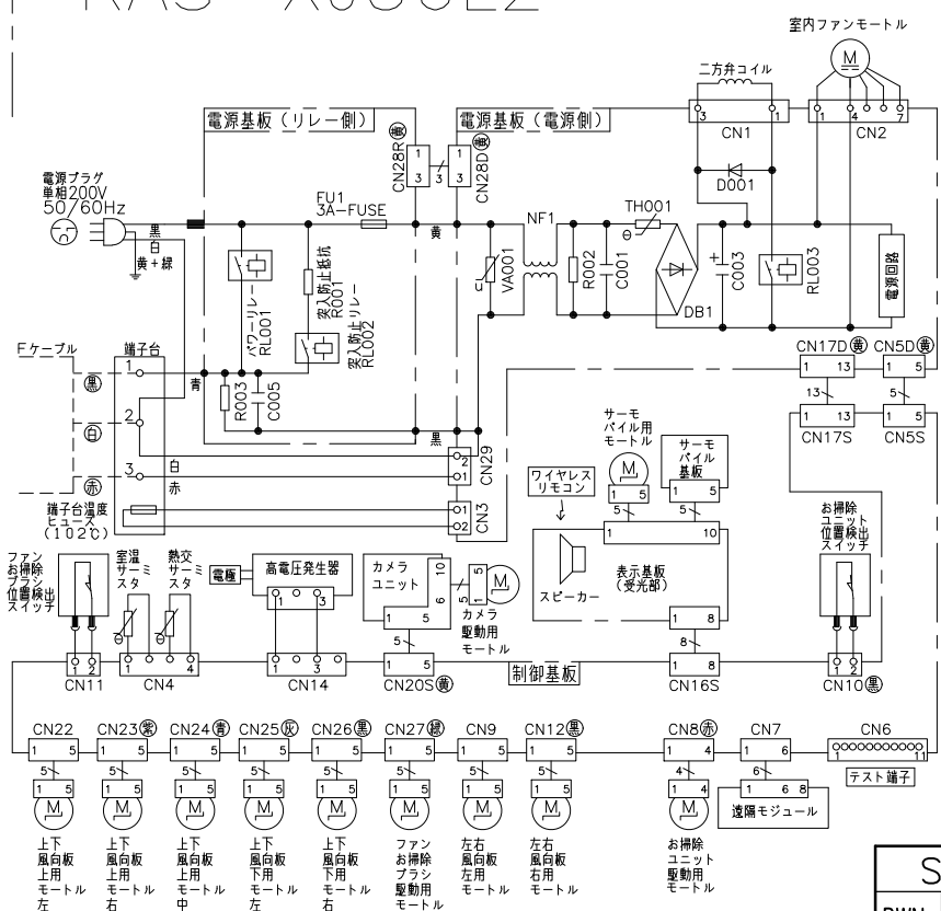
配線図 RAS-XJ56L2
